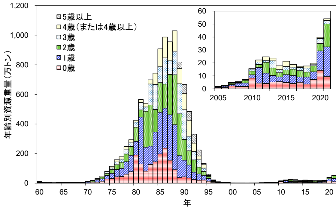
図 4-4. 年齢別資源重量の推移
