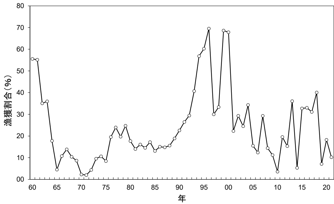
図 4-8. 漁獲割合の推移
