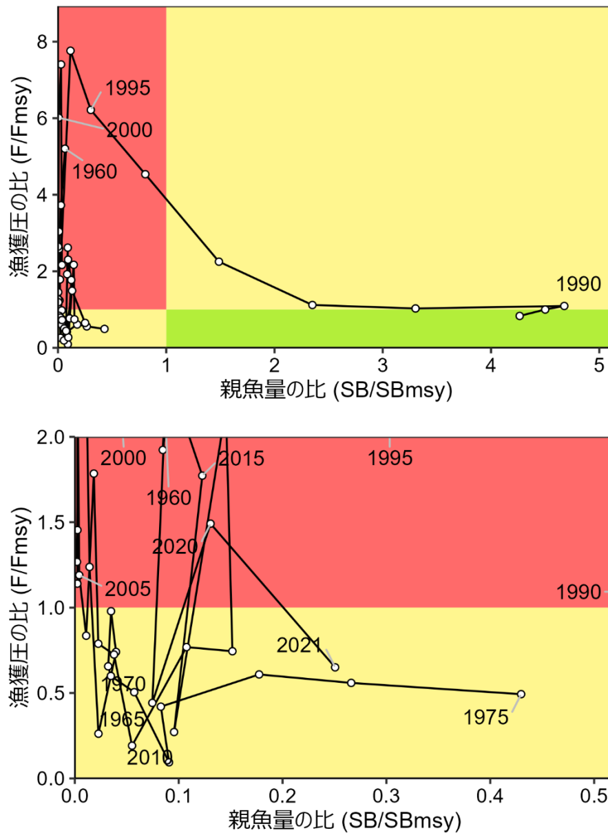
図 4-13. 最大持続生産量 MSY を実現する親魚量(SBmsy)と MSY を実現する漁獲圧(Fmsy) に対する、過去の親魚量および漁獲圧の関係(神戸プロット)とその拡大図 SBmsy および Fmsy は通常加入期(1960～1975 年および 1988～2017 年)を仮定した場合の値であり、親魚量と漁獲圧のプロットも上記の期間に限定している。
