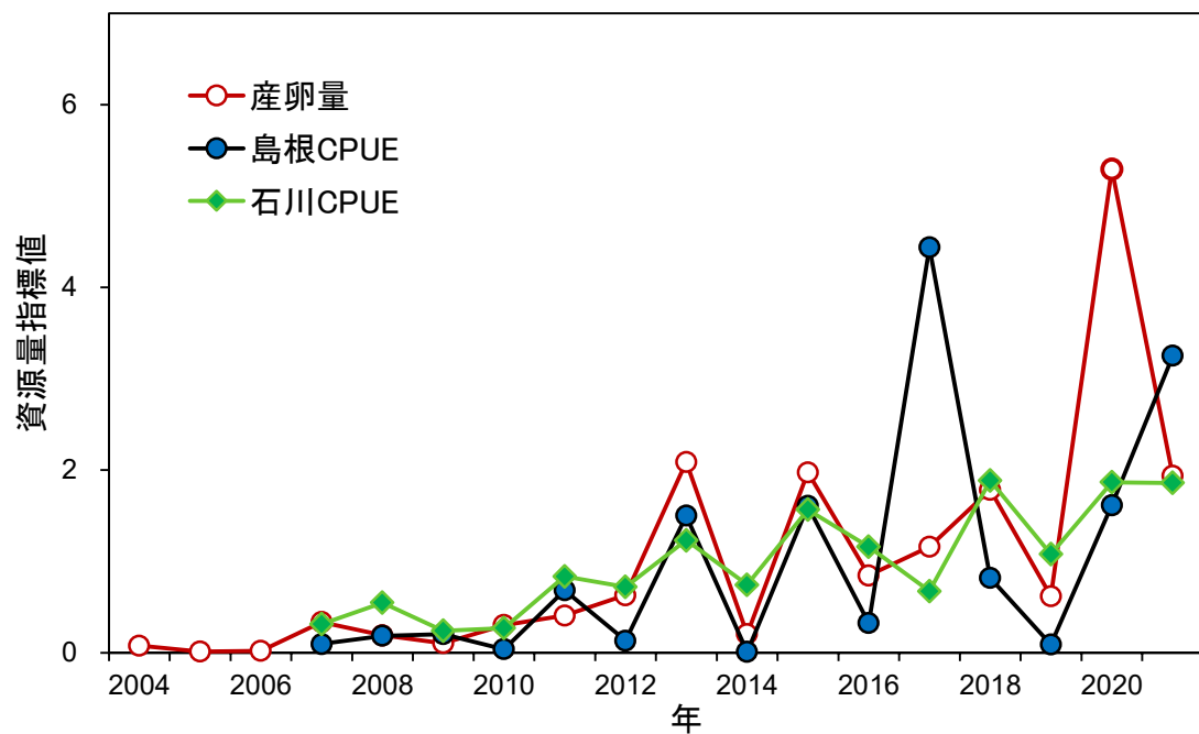
図 4-1. 資源量指標値の推移（平均値で割って規格化した数値）
