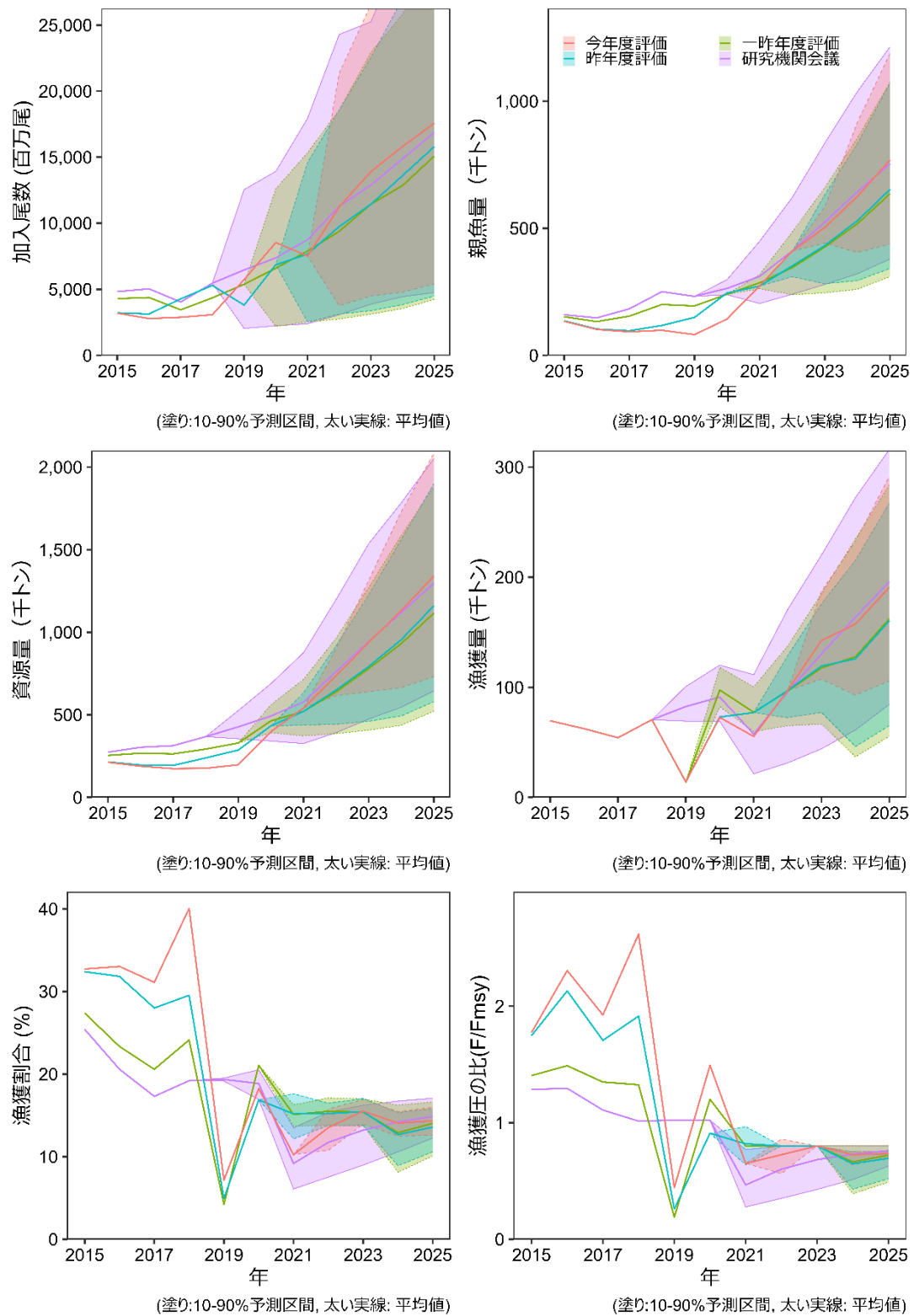
補足図 7-1. 加入尾数、親魚量、資源量、漁獲量、漁獲割合、漁獲圧の比の将来予測結果 (紫：2019 年度資源評価に基づく研究機関会議予測、緑：2020 年度資源評価、青：2021 年度資源評価、赤：今年度資源評価)
