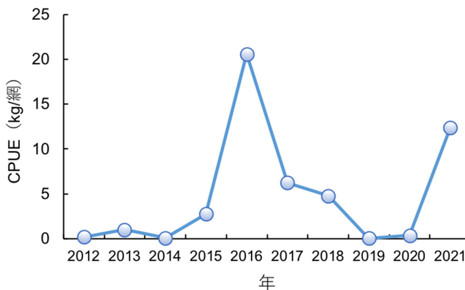
補足図4-1. 九州北西沖合域におけるマイワシのCPUE
