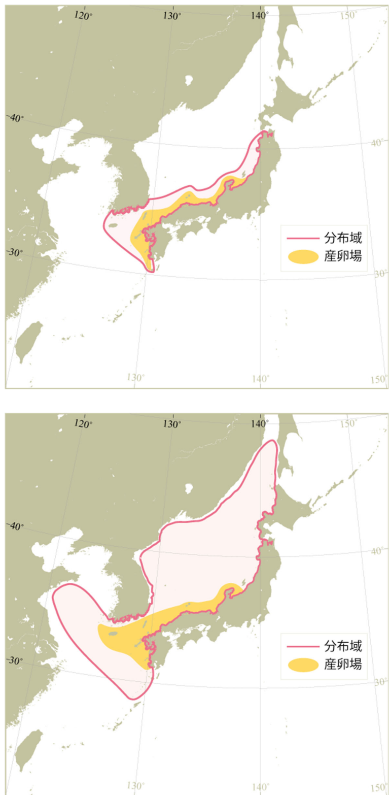
図 2-1. マイワシ対馬暖流系群の分布・回遊および生活史と漁場形成模式図(上:低水準期、 下:高水準期)
