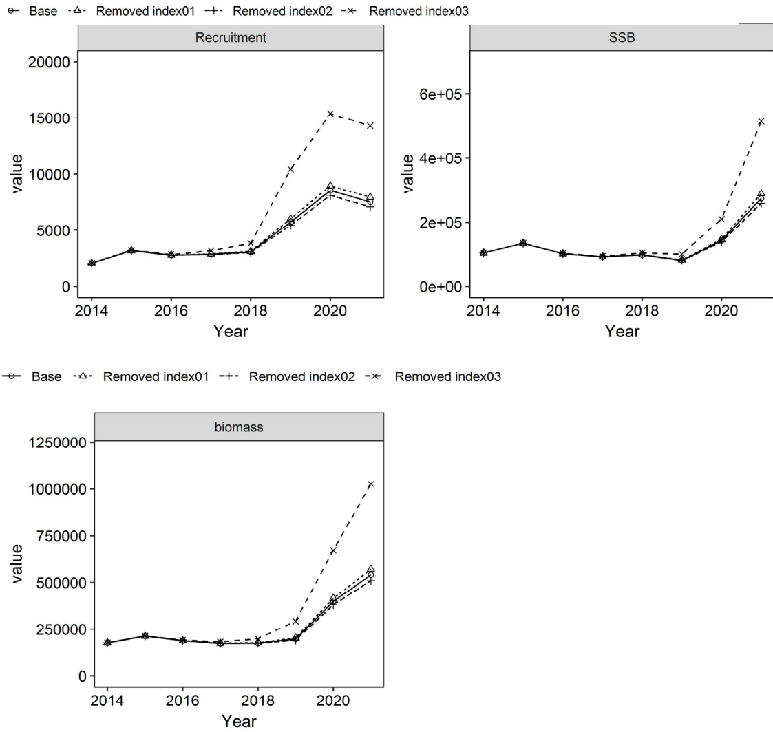
補足図 2-2. チューニング VPA のモデル診断 加入量と親魚量、資源量のジャックナイフ解析 指標値 (index 01: 島根標準化 CPUE、02: 産卵量、03: 石川 CPUE)
