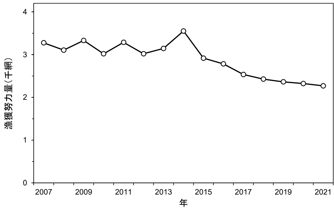
図 3-3. 島根県籍中型まき網船団の漁獲努力量（網数）の推移
