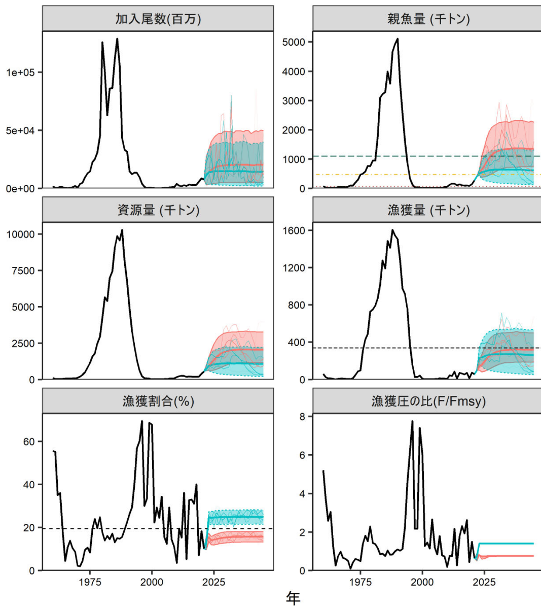
図 5-3. 漁獲管理規則を用いた将来予測(赤線)と現状の漁獲圧で漁獲を続けた場合の将来予測(緑色)
