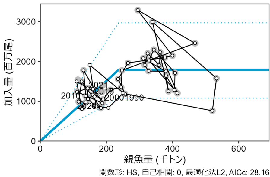
図 4-11. 親魚量と加入量の関係（再生産関係） 平成 31 年 4 月に開催された「管理基準値等に関する研究機関会議」（安田ほか 2019）で提案された再生産関係式と再生産関係のプロット（灰色の丸印）。図中の再生産関係式（青実線）の上下の点線は、仮定されている再生産関係において観察データが 90%が含まれると推定される範囲である。実線と白抜きの丸印で示したのは今年度の評価で得られた再生産関係のプロット。図中の数字は年級群を示す。
