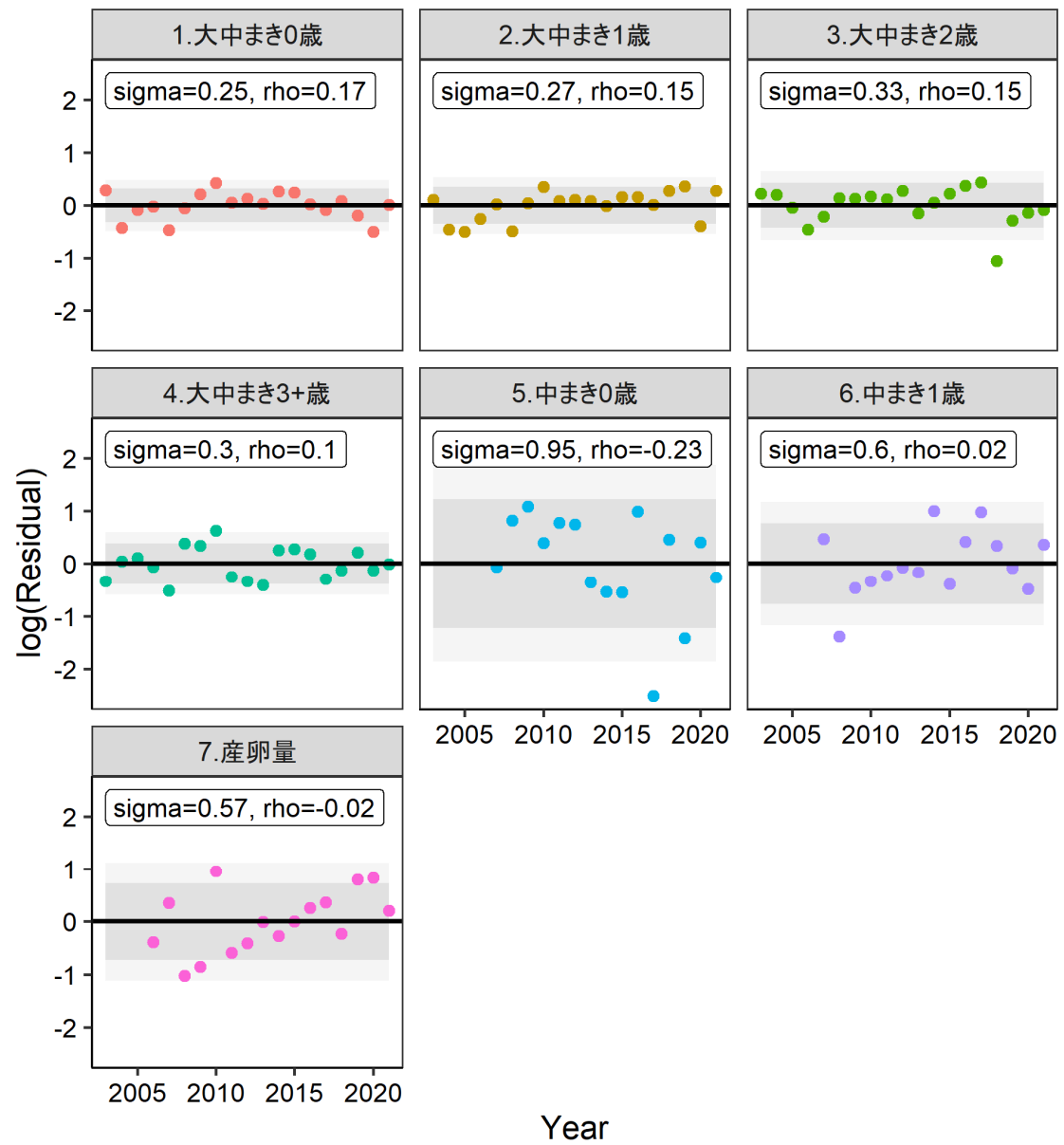
補足図 2-1. 指標値の観測値とモデルの期待値の差を示す残差プロット
