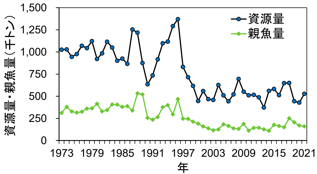
図 4-2. 資源量と親魚量の推移
