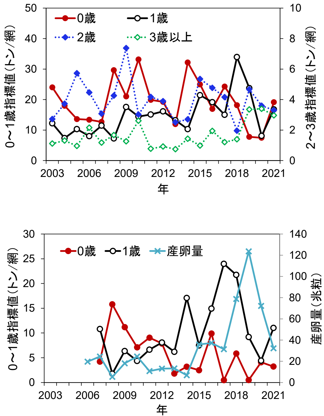
図 4-1. 東シナ海・日本海で操業する大中型まき網の銘柄別漁獲量から算出した年齢別の資源量指標値 (トン/網) の推移 (上図) と島根県籍中型まき網の豆銘柄の漁獲量と入港隻数から算定した 0 歳と 1 歳の資源量指標値 (トン/網) および産卵量による親魚量指標値 (兆粒) の推移 (下図)
