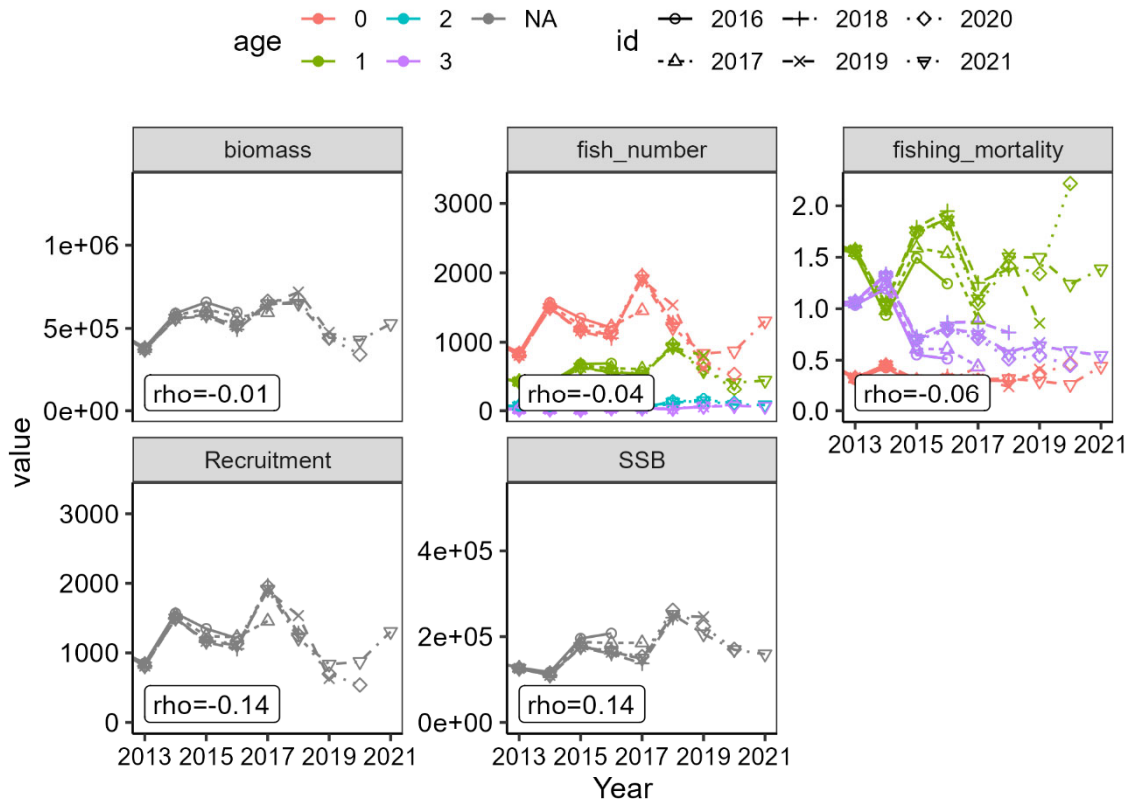
補足図 2-3. 5 年間のレトロスペクティブ解析（左上：資源量、中上：資源尾数、右上：漁獲係数、左下：加入量、中下：親魚量）
