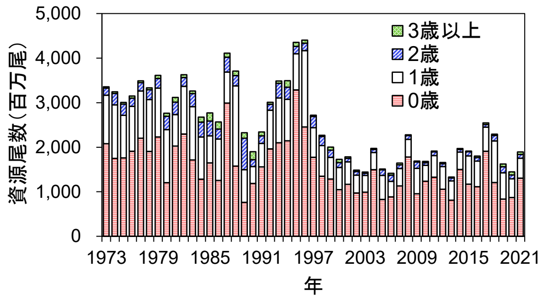
図 4-3. 年齢別資源尾数の推移
