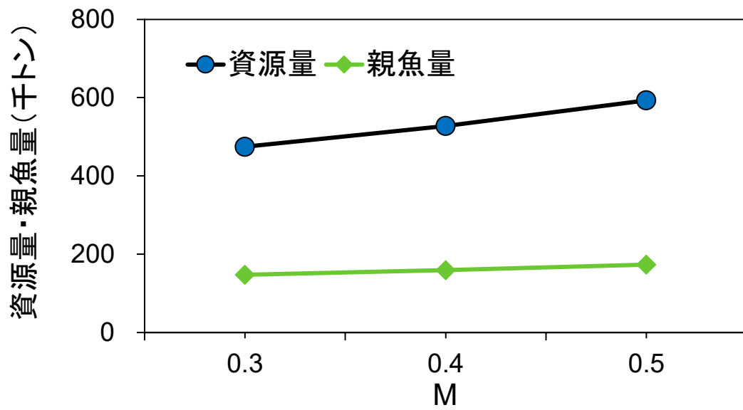
図 4-6. 2021 年の資源量と親魚量の推定に対する自然死亡係数 M の影響
