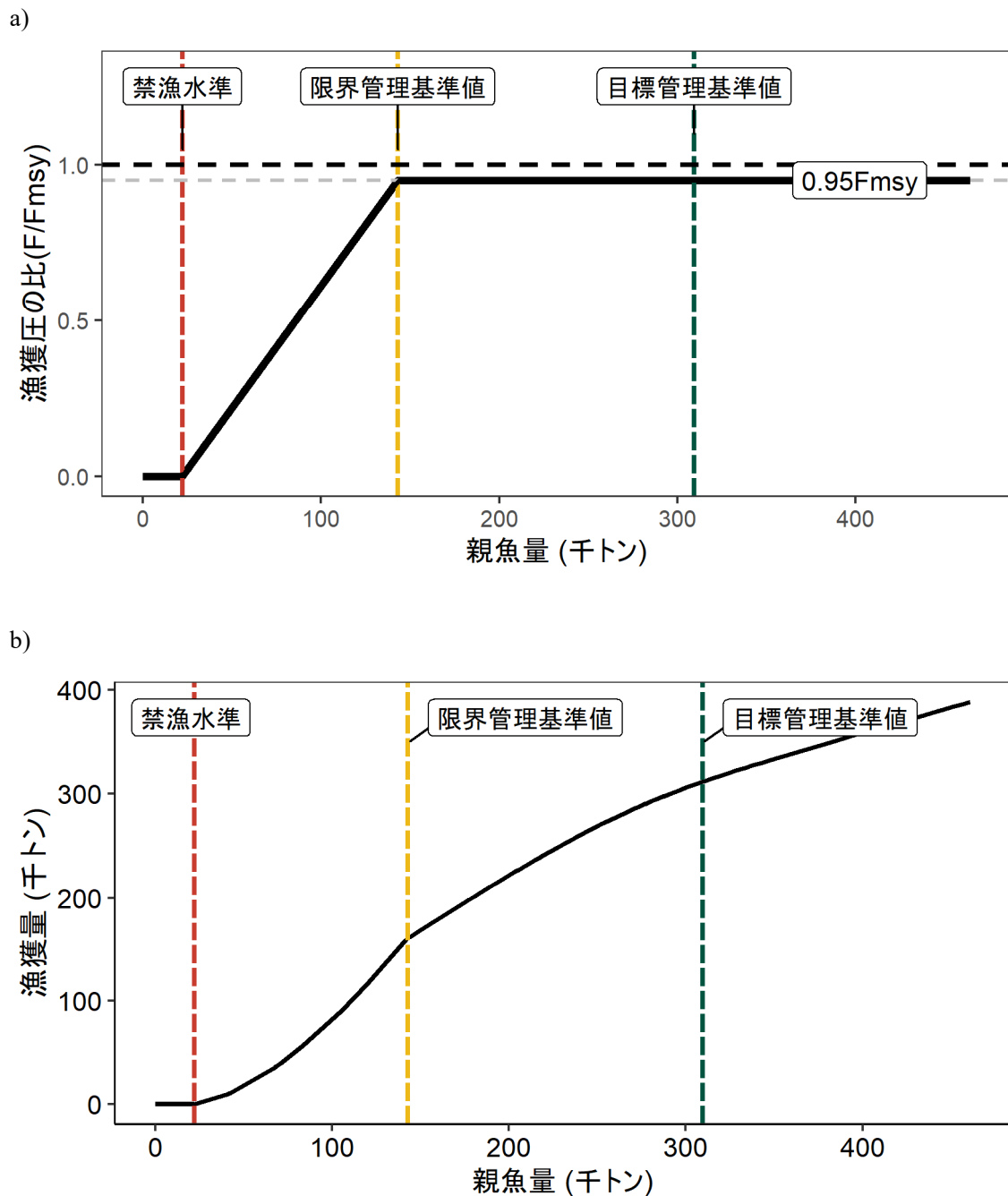
図 5-1. 漁獲管理規則（調整係数 \beta=0.95 の場合） 目標管理基準値（ SB_{target} ）はホッケ-スティック型再生産関係に基づき算出した SB_{msy} である。限界管理基準値（ SB_{limit} ）および禁漁水準（ SB_{ban} ）にそれぞれ標準値を用いている。黒破線： F_{msy} 、灰色破線： 0.95F_{msy} 、黒太線： HCR 、赤破線：禁漁水準、黄色破線：限界管理基準値、緑色破線：目標管理基準値を示す。a) は縦軸を漁獲圧にした場合、b) は縦軸を漁獲量で表した場合である。b) については、漁獲する年の年齢組成によって漁獲量は若干異なるが、ここでは平衡状態における平均的な年齢組成の場合の漁獲量を示した。
