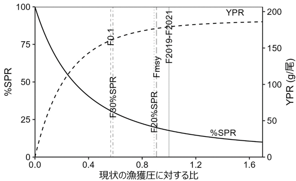
図 4-10. 現状の漁獲圧（F2019-2021）に対する YPR と%SPR の関係
