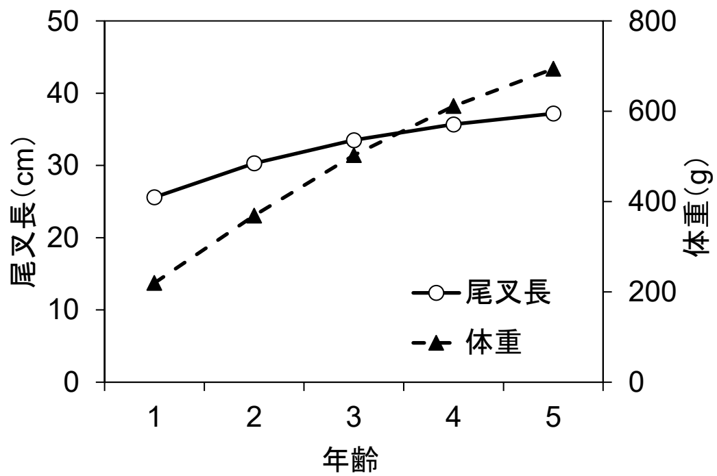
図 2-2. 年齢と成長
