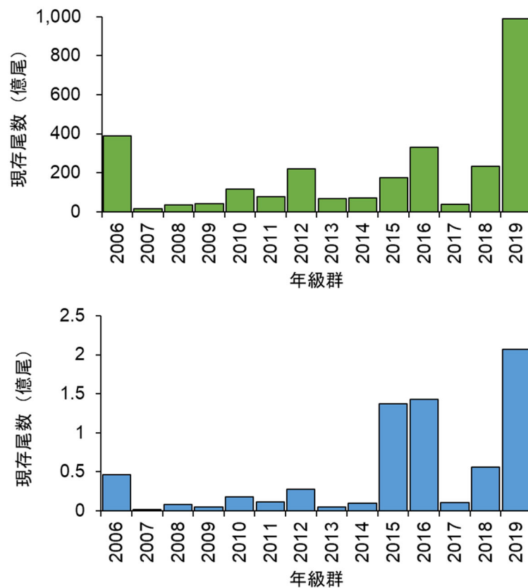
図 4-2. 加入量指標値の推移 上図は仔稚魚分布調査による 0 歳現存尾数推定値、下図は未成魚分布調査による 1 歳現存尾数推定値である（稚内・中央・函館水産試験場（2022）の図を改変）。
