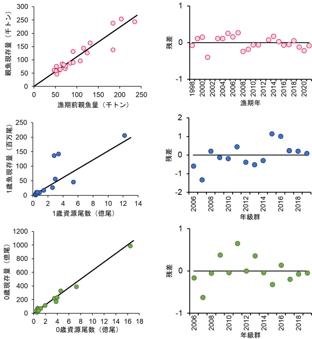
補足図 2-1b. VPA で推定された親魚量や資源尾数と各調査の現存量推定値との関係(左)
