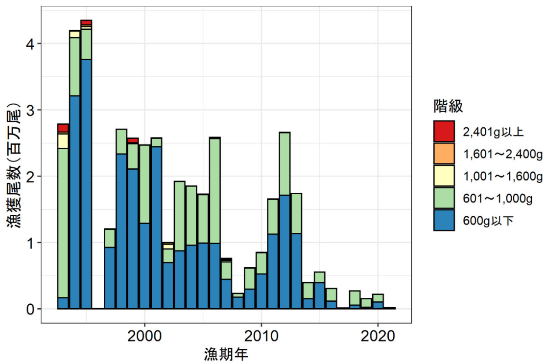
図10. 九州主要港に水揚げされたサワラの体重別漁獲尾数（漁期年は11月～翌年4月）
