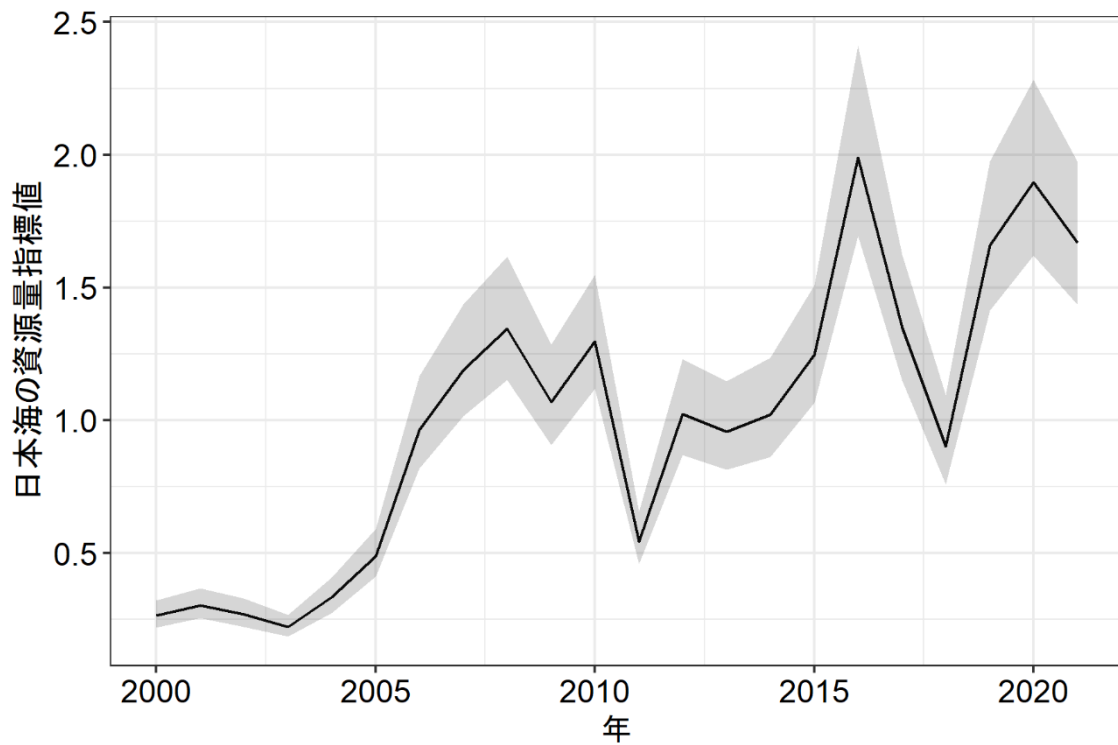
図9. 日本海における資源量指標値（定置網標準化 CPUE）と 95%信頼区間（灰色）の推移
