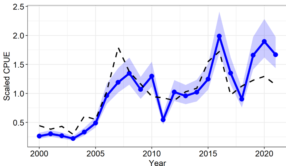
補足図 3-1. 平均値で規格化した 95%信頼区間付き標準化 CPUE (青) およびノミナル CPUE (破線)
