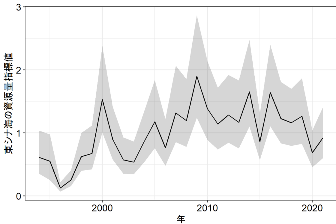
図 8. 東シナ海における資源量指標値（まき網標準化 CPUE）と 95%信頼区間（灰色）の推移
