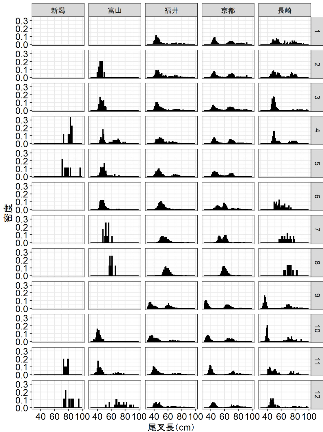
図 11. 新潟県、富山県、福井県、京都府、長崎県におけるサワラの 2021 年月別尾叉長組成（測定尾数が 5 個体以上の月を表示）
