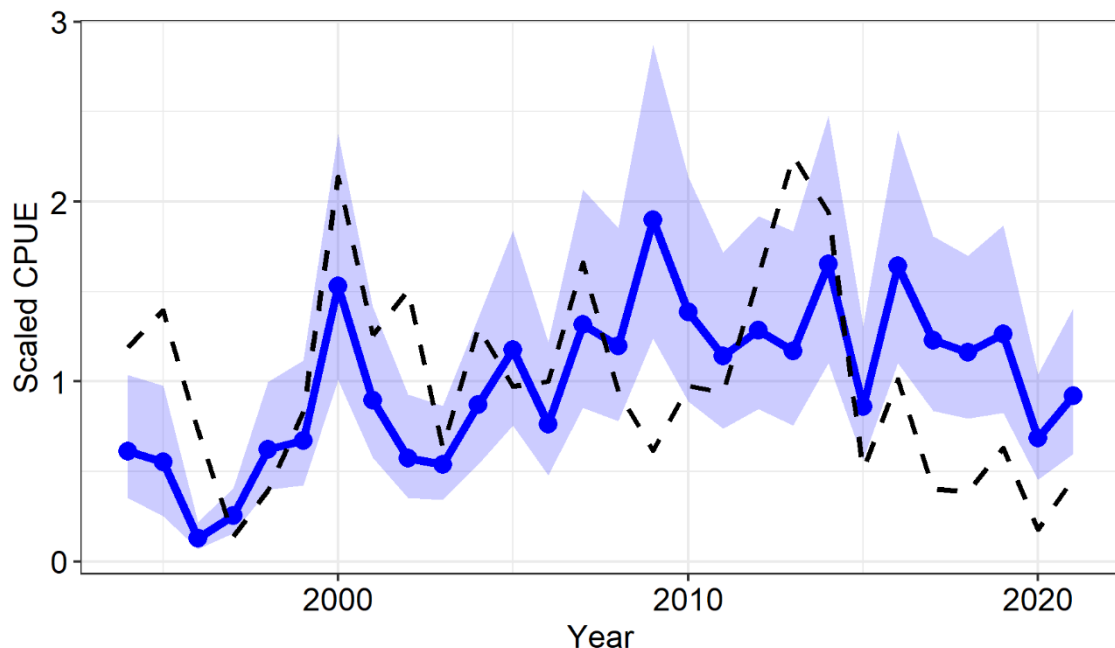
補足図 2-1. 平均値で規格化した 95%信頼区間付き標準化 CPUE (青) およびノミナル CPUE (破線)
