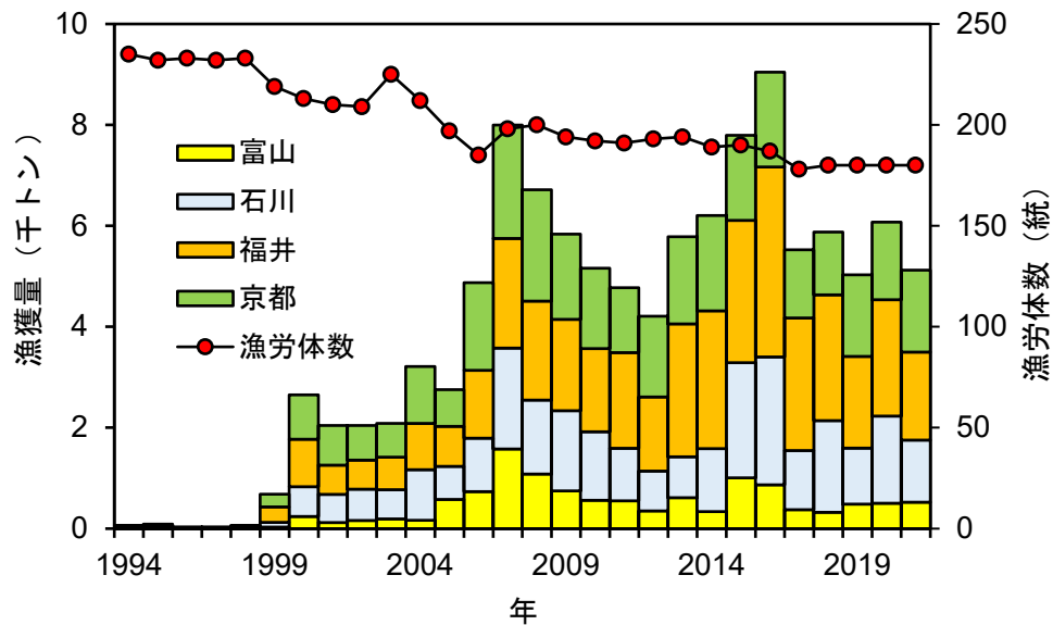
図 6. 日本海（富山県・石川県・福井県・京都府）におけるサワラ漁獲量および大型定置網の合計漁労体数（統）（2021 年漁獲量は暫定値、2019 年～2021 年の漁労体数は 2018 年の確定値）
