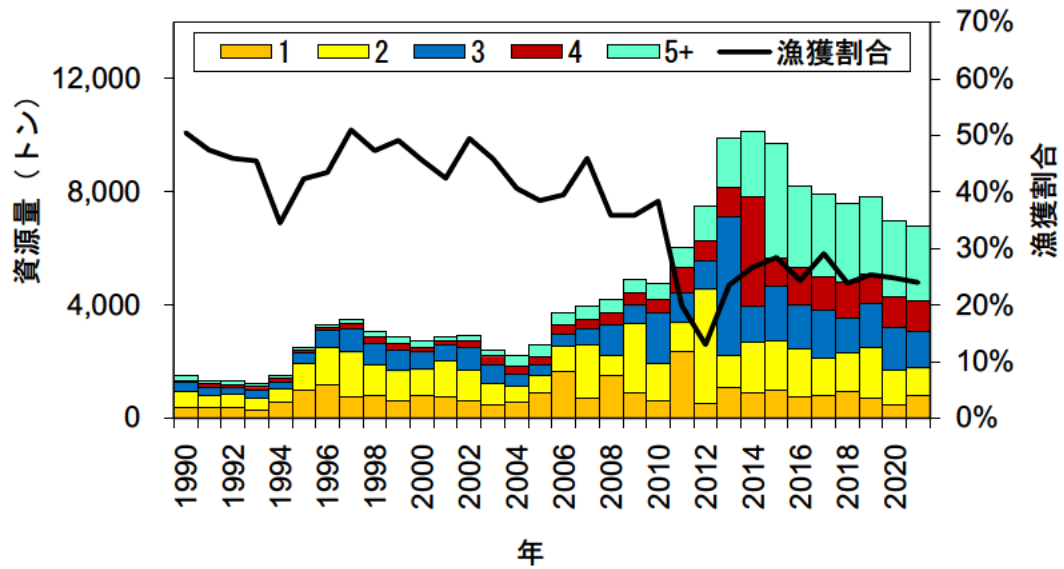
補足図 2-3. 雌雄別に推定した推定資源量と漁獲割合の推移 推定資源量は年齢別に示した。
