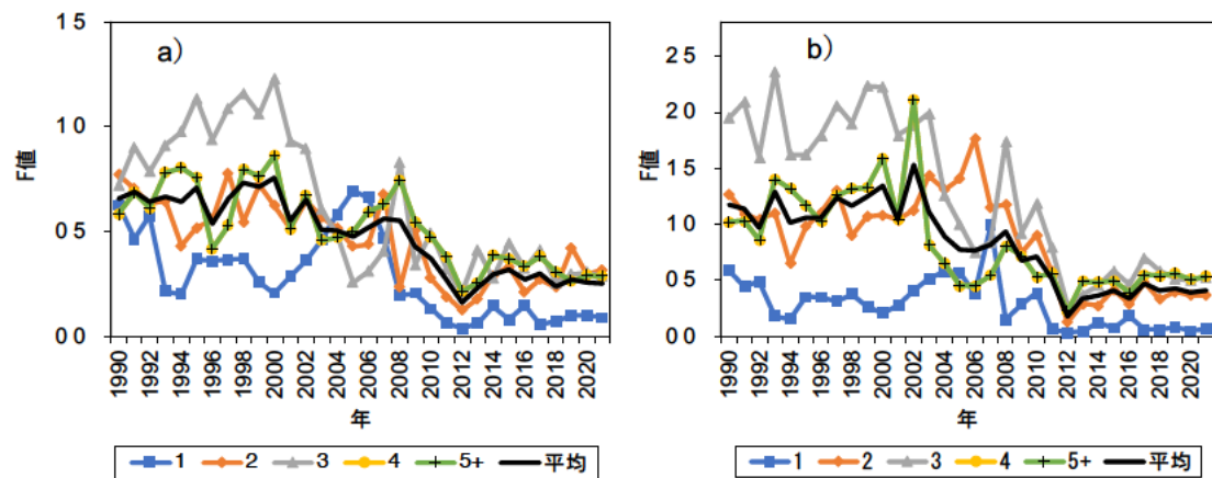
補足図 2-7. 雌雄別に推定した a) 雌、b) 雄の F 値の推移 年齢別および年齢の平均 F 値を示した。
