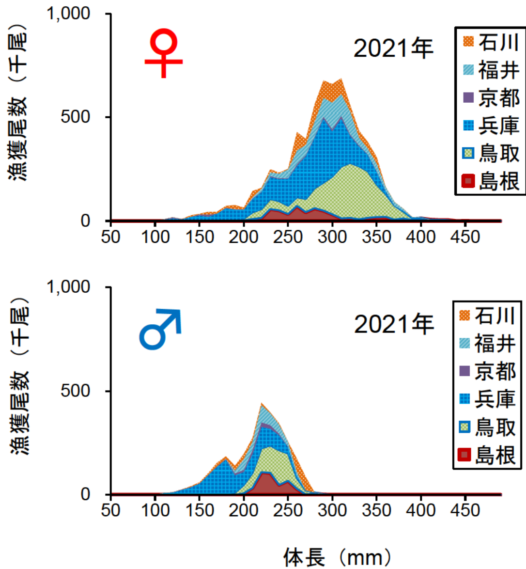
図7. 日本海西部におけるアカガレイの漁獲物の雌雄別および府県別の体長組成 兵庫県では銘柄－体長 key の更新が不十分な市場で小型個体が過大に計算されている可能性がある。
