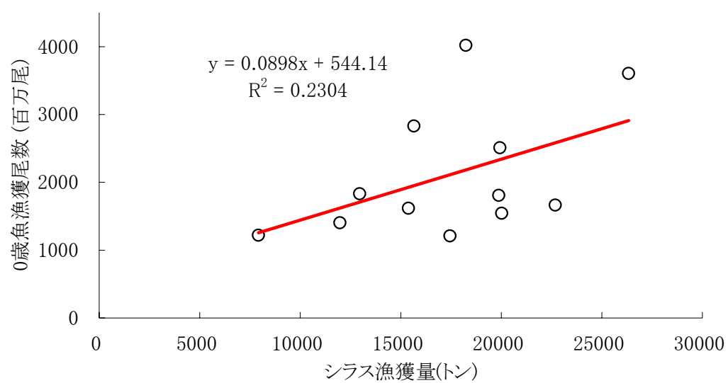
図17 1994～2005年におけるカタクチイワシ太平洋系群の0歳魚漁獲尾数(百万尾)とシラス漁獲量(神奈川～宮崎 トン)との関係
