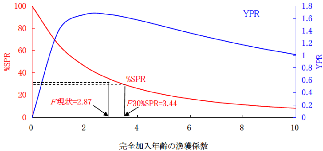
図15 カタクチイワシ太平洋系群の完全加入年齢の漁獲係数( F )と%SPR、YPRの関係 (1歳魚の F は完全加入年齢の F に0.47を乗じた値に相当する)
