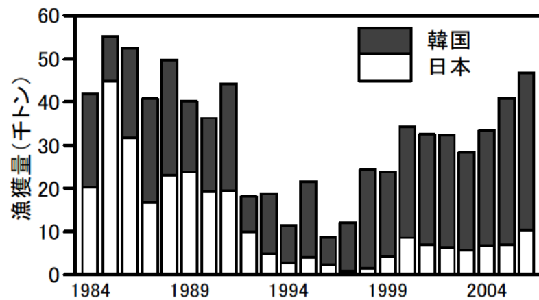
図 4. サワラ東シナ海系群の日本および韓国の漁獲量
