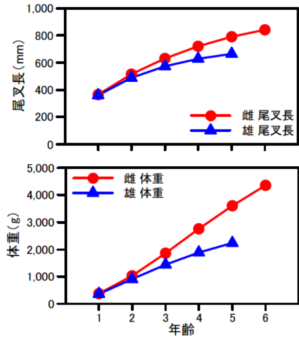
図 2. サワラ東シナ海系群の成長
