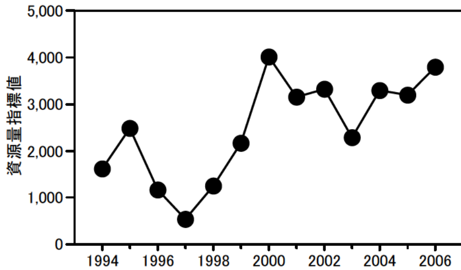
図 7. サワラ東シナ海系群の資源量指標値の推移
