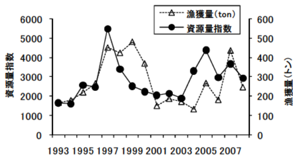
図 12. 日本海における 1～2 月の沖合底びき網（1 そうびき）によるマダラの漁獲動向（暫定版）
