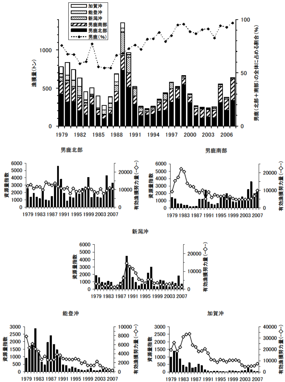
図 10. 沖合底びき網（1 そうびき）によるマダラの海区別の漁獲動向 能登沖と加賀沖の資源量指数のスケールが、他の海区の 1 / 2 であることに注意 能登沖と加賀沖の有効漁獲努力量のスケールが、他の海区と異なっていることに注意 海区：日本海区水産研究所（2007）に基づく
