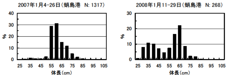
図 15. 石川県の底びき網漁船が漁獲したマダラの体長組成（対象：25cm 以上） 「日本海中部海域マダラ栽培漁業資源回復等対策事業」のデータを一部使用 ただし、全長データは桜井・福田(1984)に基づき体長に換算
