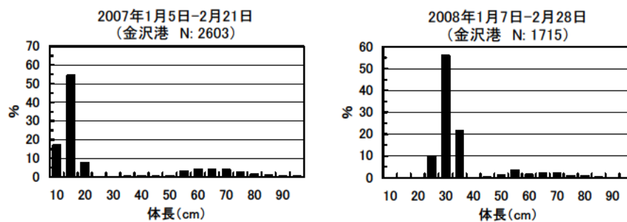
図 21. 2007～2008 年 1～2 月に石川県の底びき網漁船が漁獲したマダラの体長組成 「日本海中部海域マダラ栽培漁業資源回復等対策事業」のデータを一部使用 ただし、全長データは桜井・福田(1984)に基づき体長に換算
