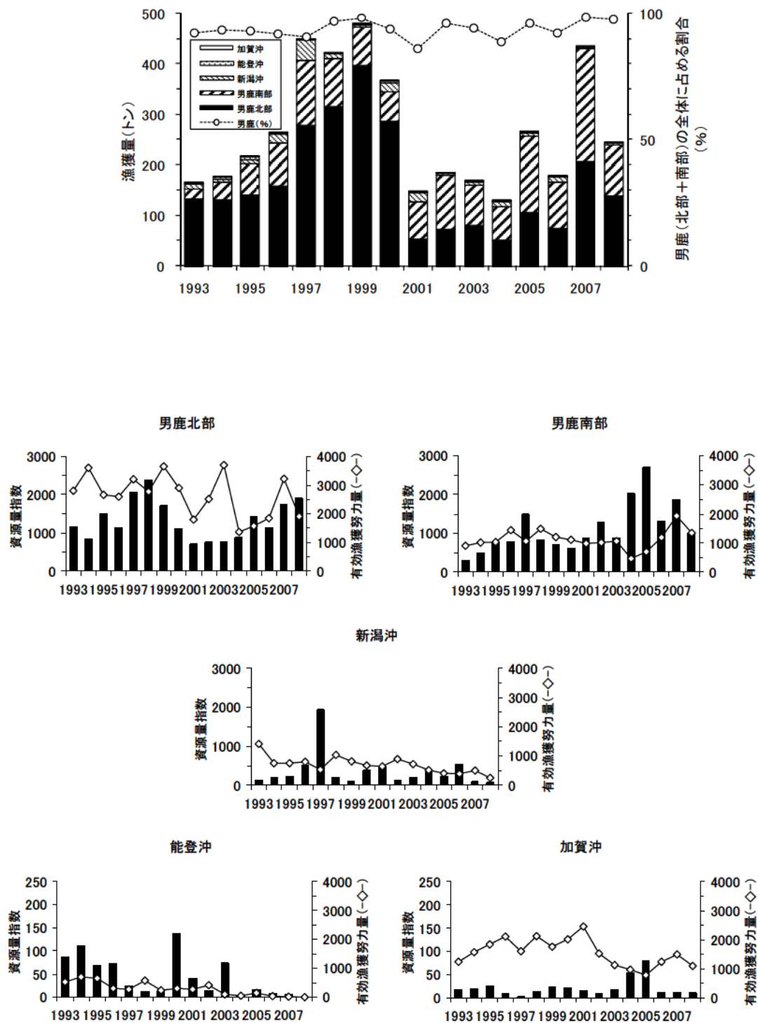
図 11. 1～2 月の沖合底びき網（1 そうびき）によるマダラの海区別漁獲動向（暫定版） ただし、2008 年の男鹿北部において、極端に漁獲量が多いまたは CPUE が高い操業結果（1 月：3 件、合計 37 トン、2 月：6 件、合計 23 トン）は計算対象外とした。 能登沖と加賀沖の資源量指数のスケールが、他の海区の 1 / 1 2 であることに注意 海区：日本海区水産研究所（2007）に基づく
