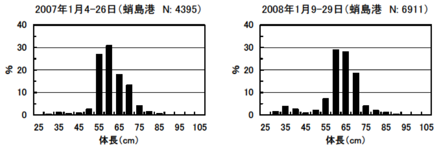
図 16. 石川県の刺網漁船が漁獲したマダラの体長組成 (対象: 25cm 以上) 「日本海中部海域マダラ栽培漁業資源回復等対策事業」のデータを一部使用 ただし、全長データは桜井・福田(1984)に基づき体長に換算
