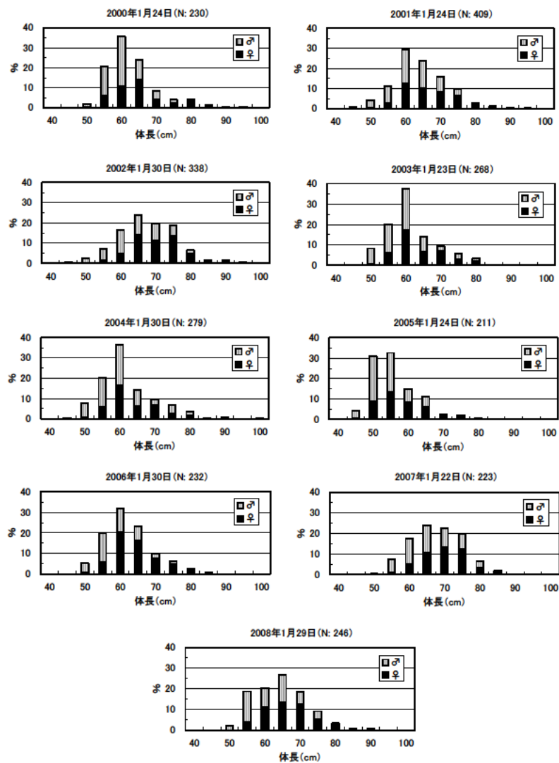
図 17. 山形県の小型底びき網漁船が漁獲したマダラの体長組成
