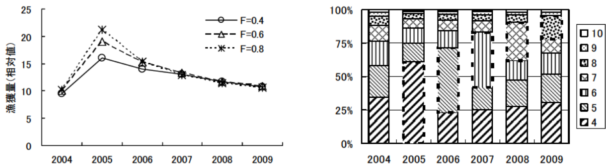
図 20. 2001 年級群マダラ当歳魚の資源個体数が他の年の 3 倍であったときに想定される 2004～2009 年の漁獲量（相対値：左図）と年齢別漁獲重量比（右図： F=0.4 ）の経年変化 自然死亡係数を 0.25、漁獲開始年齢を 4 歳、寿命を 10 歳と仮定 漁獲死亡係数（ F ）：3 種類（0.4・0.6・0.8）を仮定 右図の点線で囲まれた棒グラフは、2001 年級群に相当
