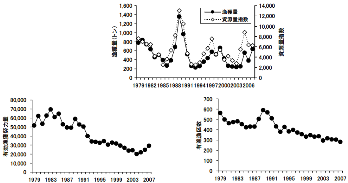
図 9. 沖合底びき網（1 そうびき）によるマダラの漁獲動向 資源量指数：各月漁区（10 分刻み）ごとの CPUE(kg/網)の総和
