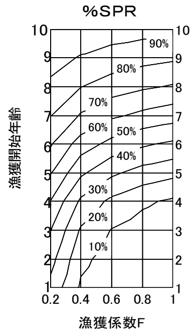
図 19. マダラの等産卵資源量図
