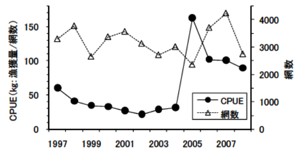
図 13. 山形県の 1～2 月の小型底びき網によるマダラの漁獲動向（漁区番号 29・135）
