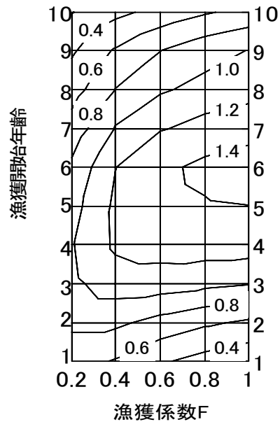
加入量あたり漁獲量(相対値)
