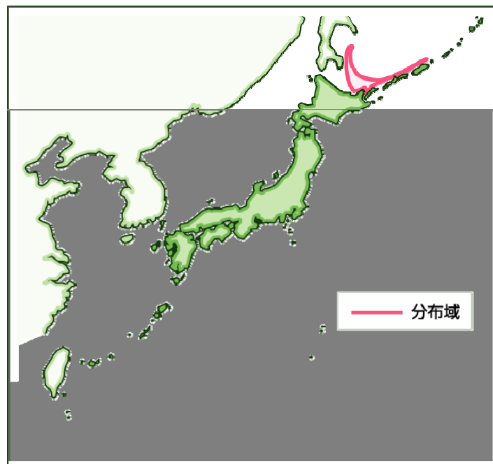
図 1. キチジ・オホーツク海系群の分布域（漁場）
