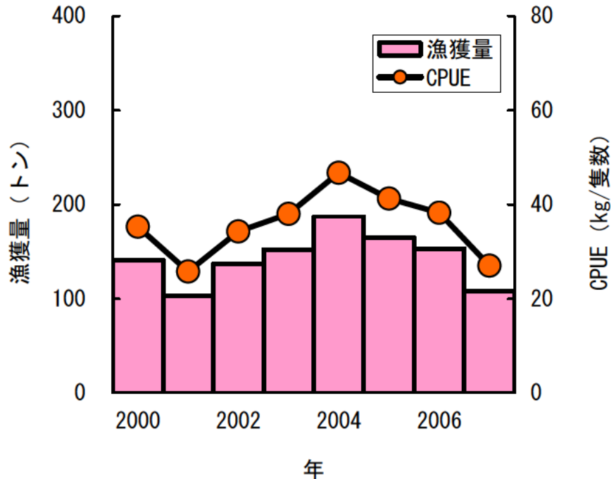
図3. オホーツク海における延縄漁業の漁獲量とCPUE（資源量指標値）の推移 （網走水産試験場資料）
