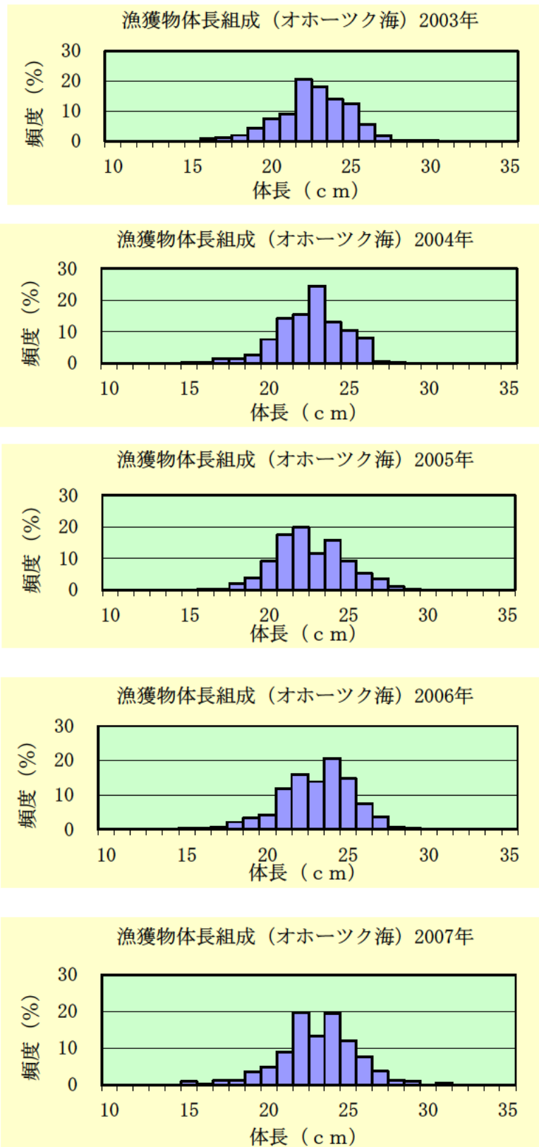
図4. キチジ・オホーツク海系群の漁獲物の体長組成 (オホーツク海における延縄漁業の漁獲物、網走水産試験場資料)
