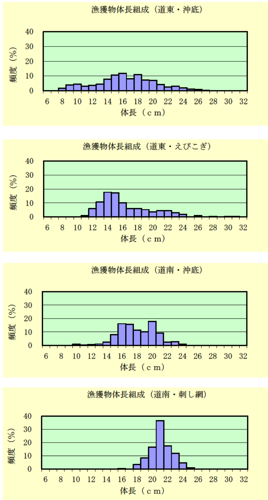
図4. キチジ道東・道南の海域別、漁業種類別の漁獲物体長組成 (2007年) (釧路水産試験場資料、栽培水産試験場資料)
