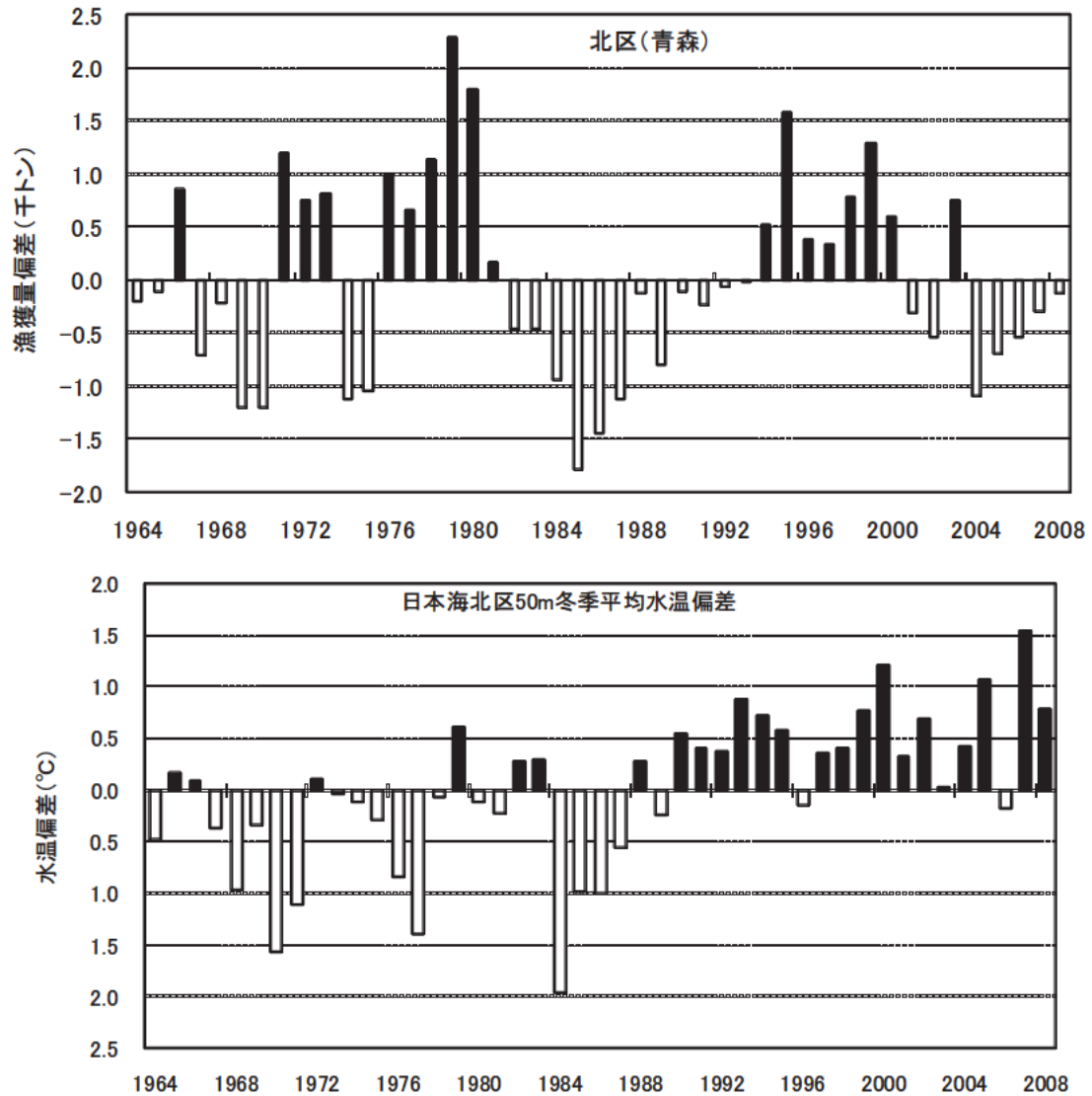
図6. 青森県におけるヤリイカ漁獲量の偏差（上）と日本海北区50m深冬季水温の偏差（下）の推移 注：偏差は各年と平年値（1964～2008年の45年平均）の差
