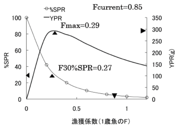
図 17. %SPR・YPR
