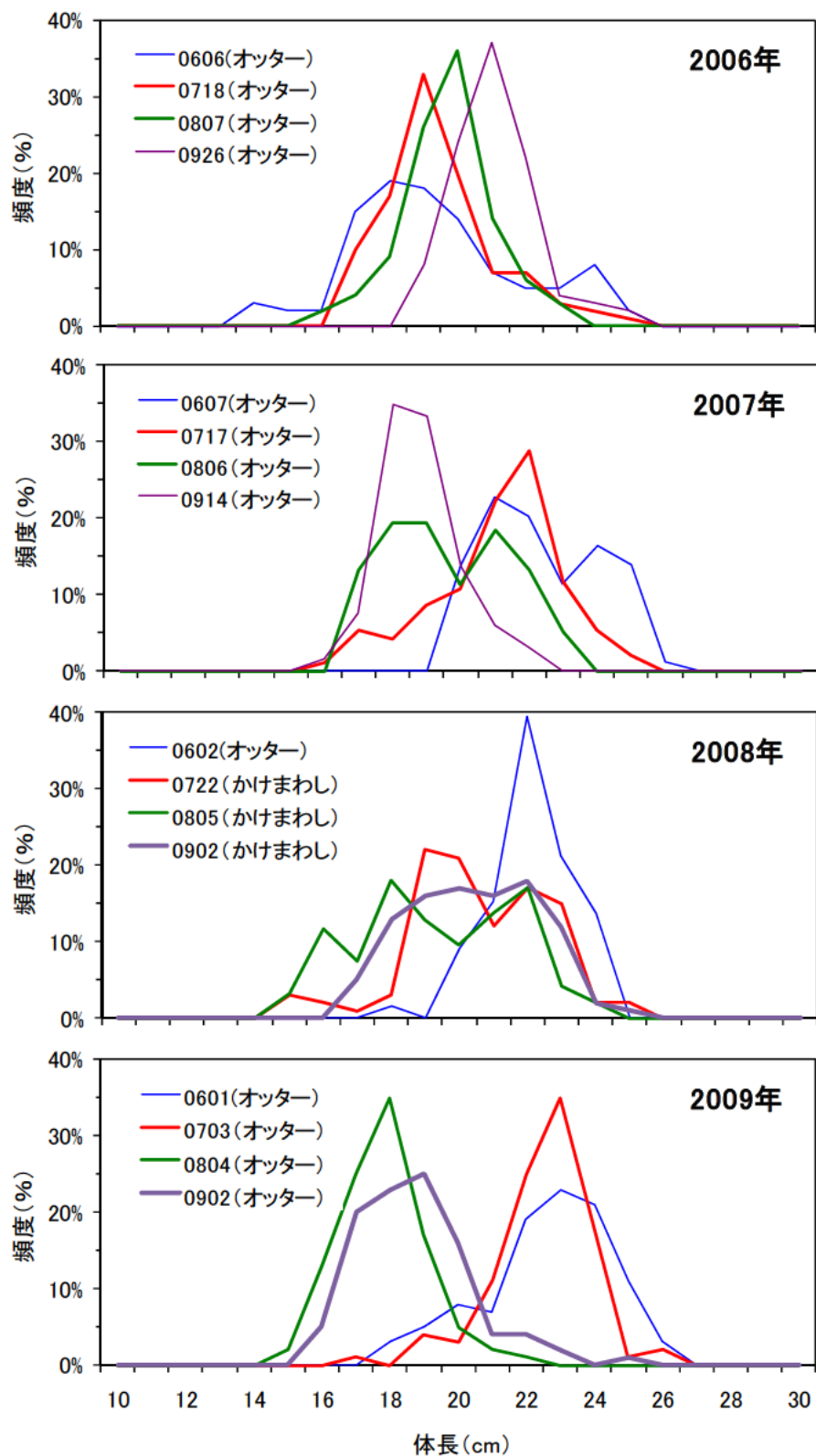
図5.宗谷海峡周辺海域において沖底（オッタートロール、かけまわし）により漁獲されたイカナゴ類の6～9月の体長組成（稚内水産試験場未発表資料）
