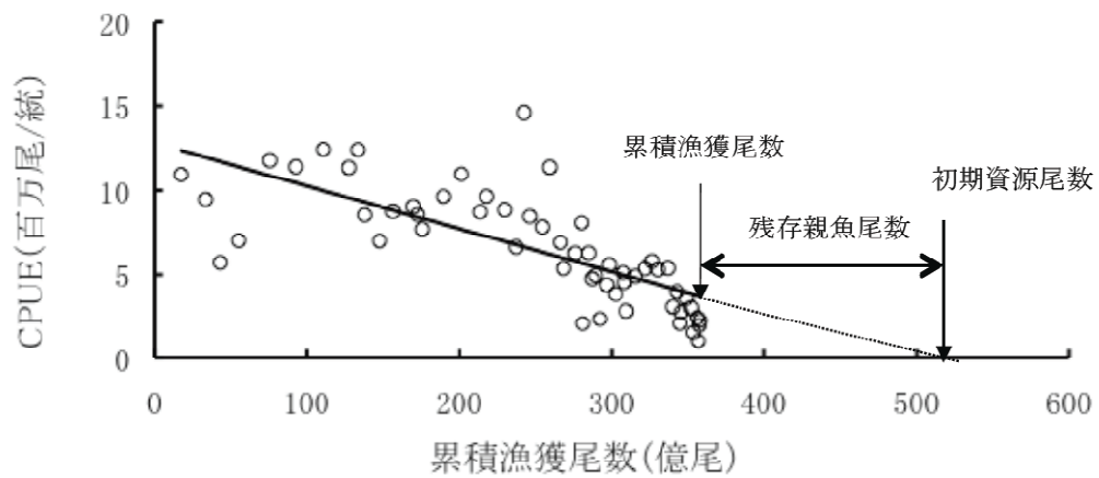
図 3. 2010 年漁期中の船びき網による累積漁獲尾数に対する CPUE の関係
