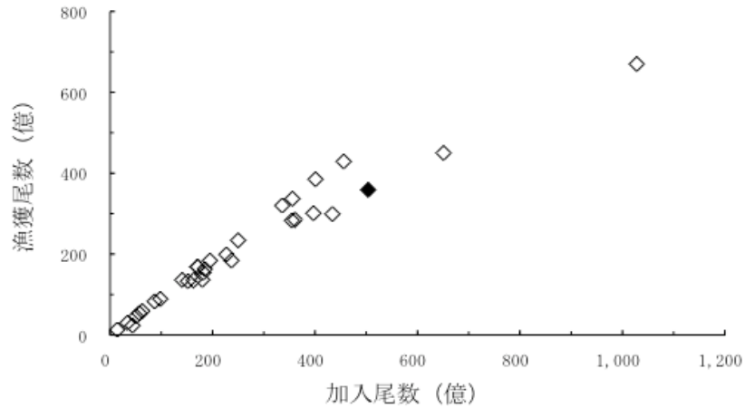
図5. 伊勢三河湾におけるイカナゴのDeLury法によって推定された0歳魚加入尾数に対する漁獲尾数の関係（1980～2010年）
