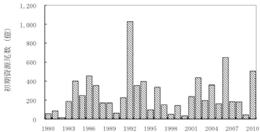
図 4. 伊勢三河湾におけるイカナゴの推定初期資源尾数の経年変化（1980 年～2010 年）
