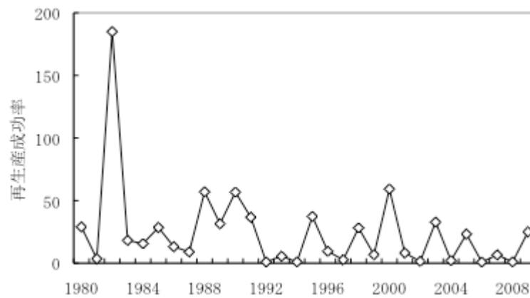
図7. 伊勢三河湾におけるイカナゴの再生産成功率（翌年の加入尾数/残存資源尾数）の経年変化（1980年～2009年）
