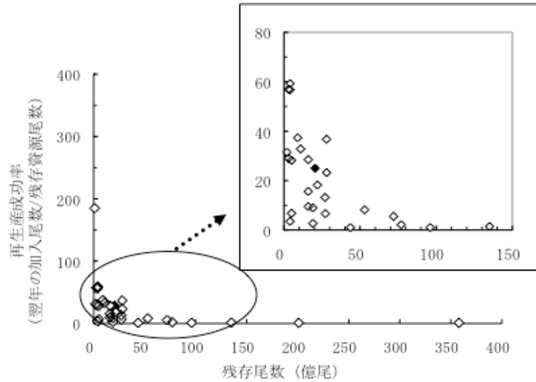
図8. 伊勢三河湾におけるイカナゴの残存資源尾数に対する再生産成功率の関係（1980年～2009年） 黒プロットは2009年のデータを示す。
