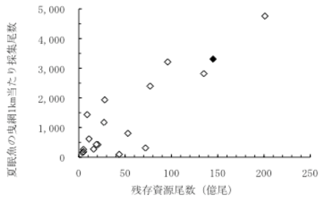
図9. 残存資源尾数に対する夏眠魚採集密度指数の関係（1993年～2010年） 黒プロットは2010年のデータを示す。
