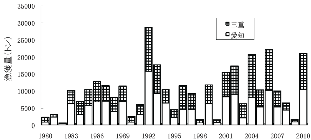
図 2. 伊勢三河湾におけるイカナゴの漁獲量の経年変化（1980 年～2008 年は農林統計確定値、2009 年は農林統計暫定値、2010 年は県データ）
