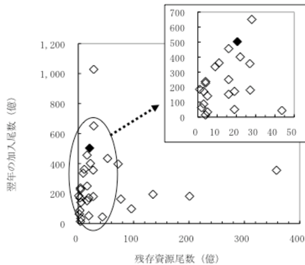
図6. 伊勢三河湾におけるイカナゴの残存資源量（取り残し0歳魚尾数）に対する、翌年0歳魚の加入尾数の関係（1980～2009年） 黒プロットは2009年のデータを示す。
