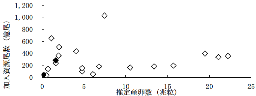
図10. 伊勢・三河湾におけるイカナゴの推定産卵数に対する、翌年の加入資源尾数の関係 (1992-2010年) ●:2008年、◆:2010年。
