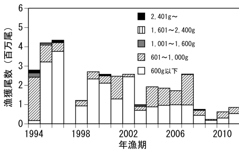
図 7. 九州主要港に水揚げされたサワラの体重別漁獲尾数
