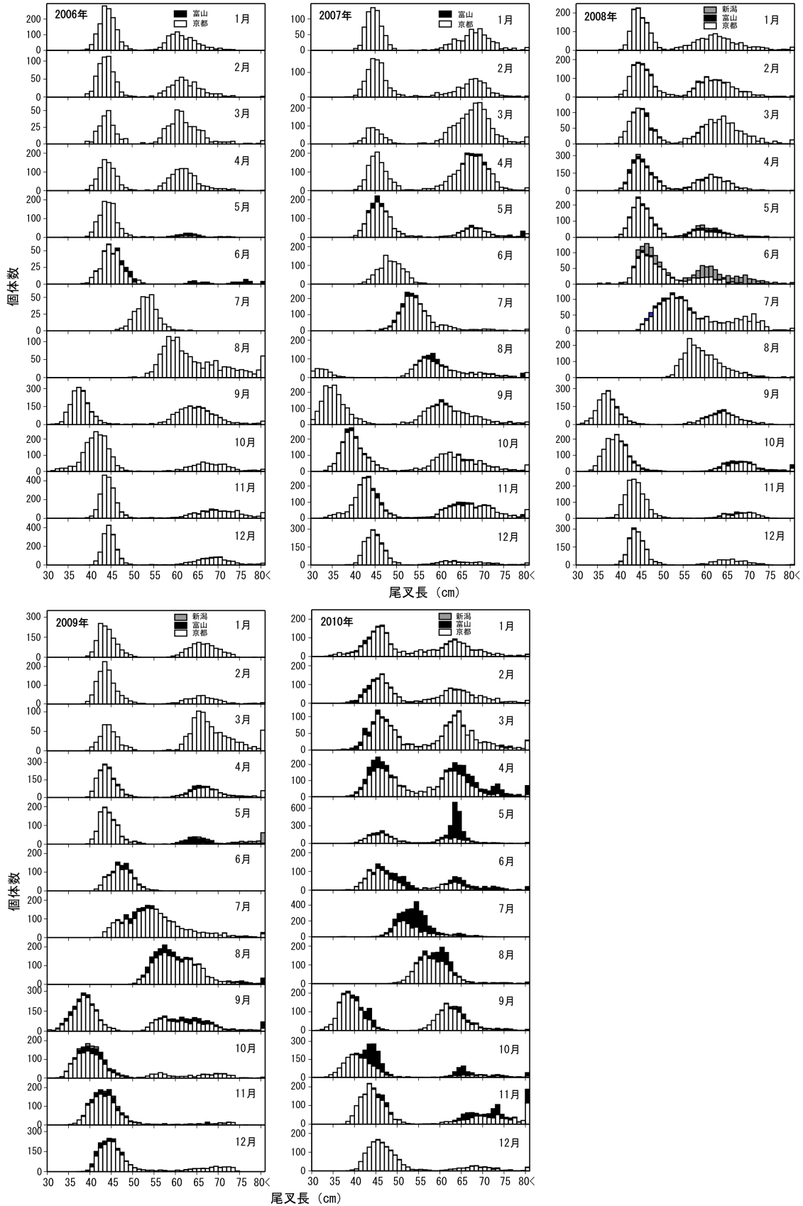
図 8. 新潟県、富山県、京都府に水揚げされたサワラの尾叉長組成
