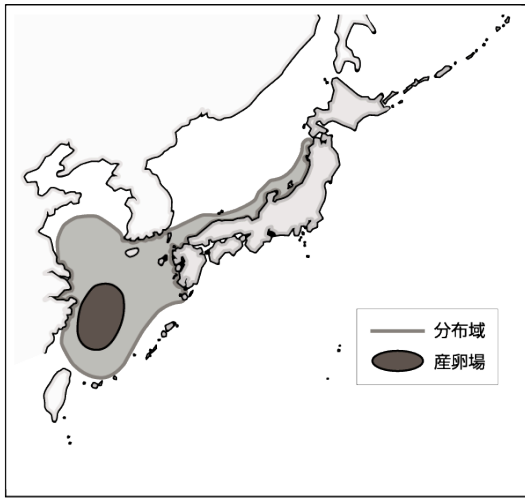
図 1. サワラ東シナ海系群の分布・回遊
