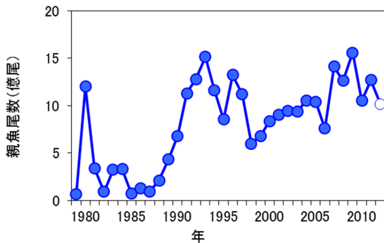
図 11. 親魚尾数の経年変化（白丸で示した 2012 年は暫定値）
