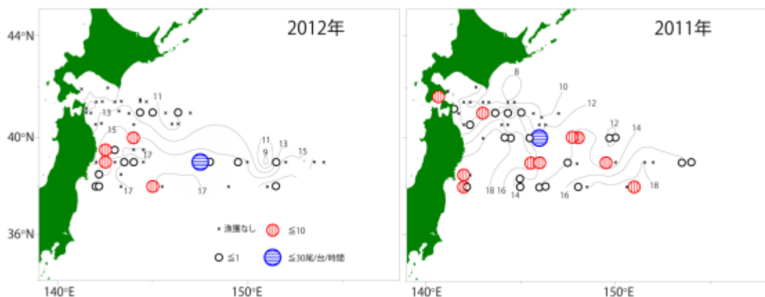
補足図 6. 2011、2012 年に実施された第1次漁場一斉調査における CPUE（釣り機1台1時間あたり漁獲尾数）の分布 ×は漁獲が無かった点、実線は海面水温の等温線。
