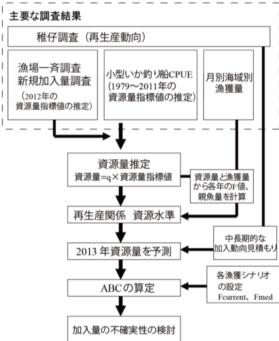
補足資料 1. データと資源評価の関係を示すフロー
