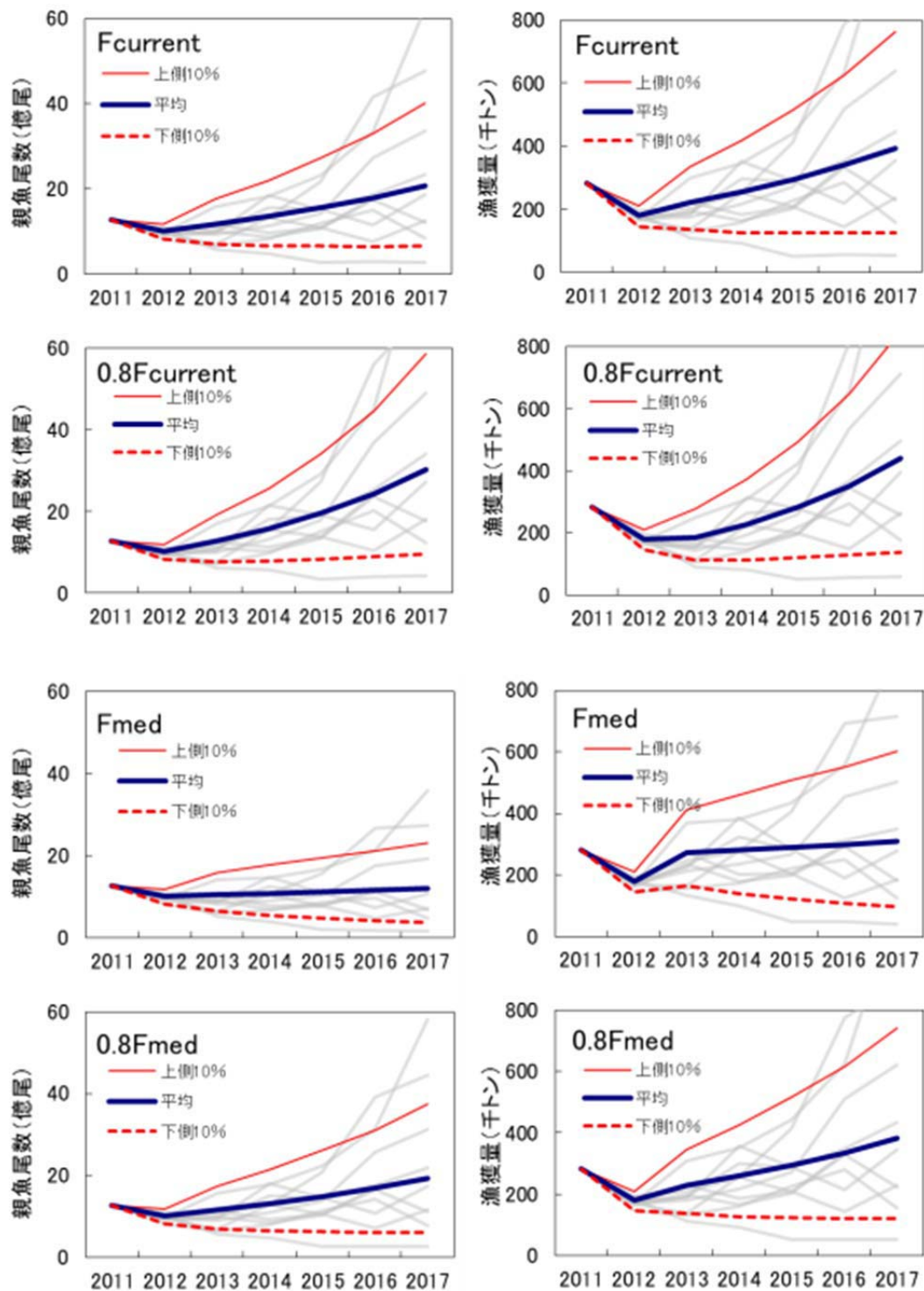
図 18. Fcurrent、0.8Fcurrent、Fmed、0.8Fmed で漁獲した場合の RPS の変動を考慮した 20,000 回のシミュレーションによる親魚尾数 (億尾) と漁獲量 (千トン) の将来予測 灰色の線は、20,000 回の試行のうち、任意の 10 回の試行の各推移、太い実線、細い実線および破線は、それぞれ 20,000 回の試行による平均値、上側 10% および下側 10% 点を示す。
