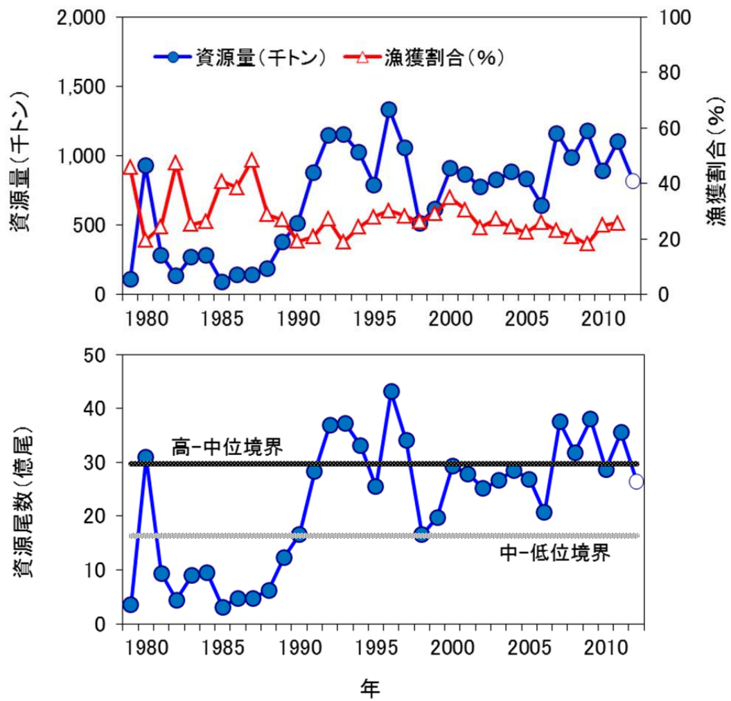
図 10. 資源量と漁獲割合（上図）と資源尾数と資源水準の境界（下図） （白丸で示した 2012 年は加入量モデルからの推定値）
