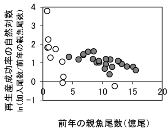
図 16. 親魚尾数と再生産成功率の関係 白丸は寒冷期（1981～1989 年）、黒丸は温暖期（1990～2012 年）。
