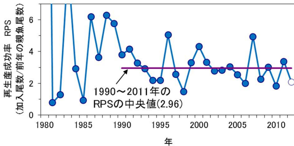
図 14. 再生産成功率 (RPS、加入尾数/前年の親魚尾数) の経年変化 (白丸で示した 2012 年は暫定値)
