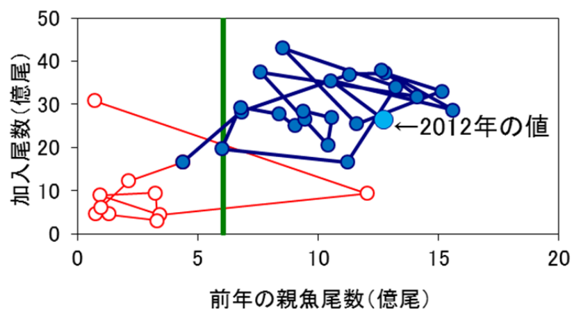
図 15. 再生産関係 赤丸は寒冷期 (1980~1989 年)、青丸は温暖期 (1990~2012 年)。 2012 年の値は暫定値。図中の縦線は B_{limit} (6.0 億尾) を示す。
