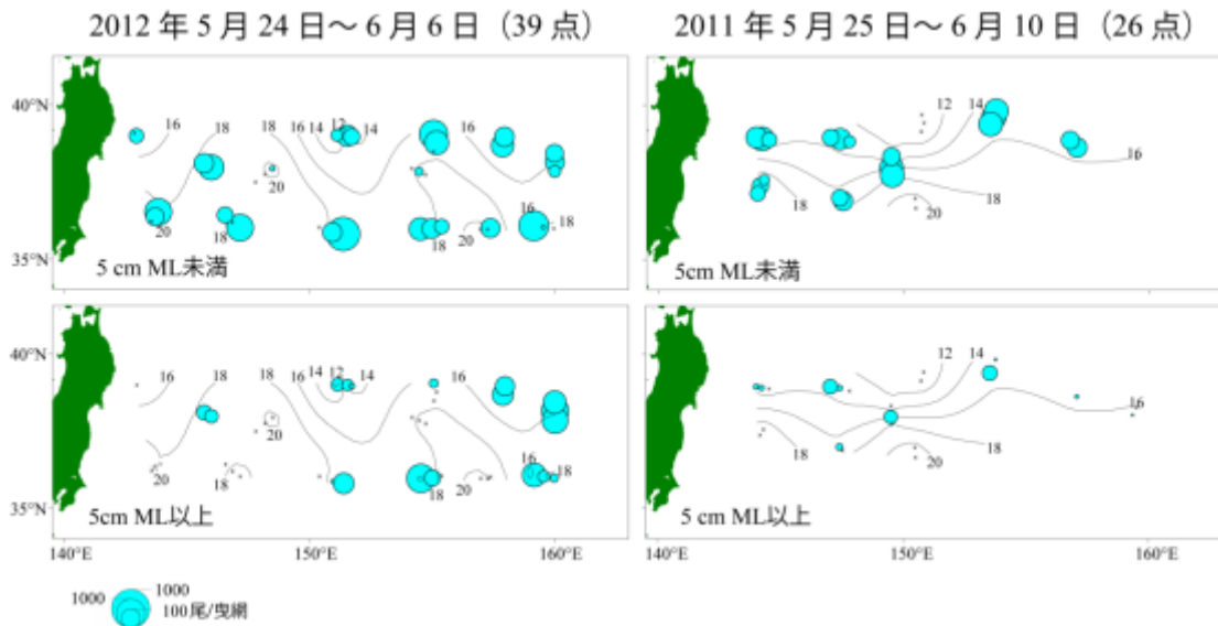
補足図 4. 2011 年、2012 年 5～6 月に表層トロールネットで漁獲した幼体の水平分布と海面水温（×は採集がなかった調査点）
