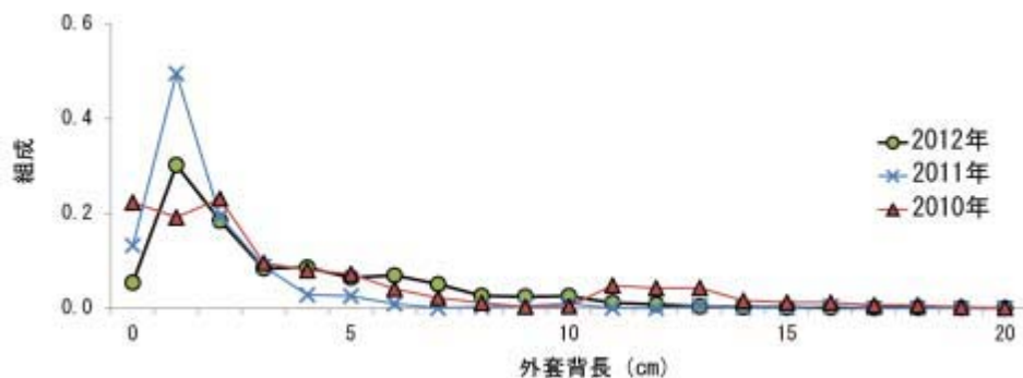
補足図 5. 表層トロールネットで採集された幼体の外套背長組成 （2012 年の値は速報値）
