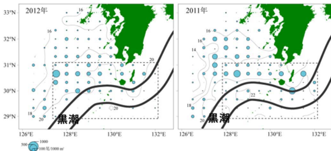
補足図 3. 2011 年、2012 年 1 月下旬～2 月下旬の東シナ海周辺海域で採集されたスルメイカ幼生の水平分布、海面水温（細実線）および黒潮流路（太実線矢印） 図内の点線で囲まれた海域は 1996 年以降、継続的に調査を実施している海域を示す。 黒潮流路は、海洋速報（海上保安庁 2011、2012）を引用。
