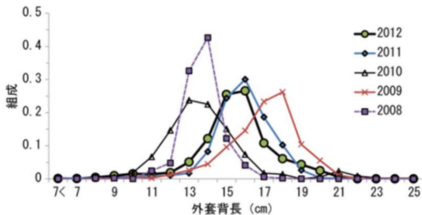
図 9. 漁場一斉調査結果による外套背長組成
