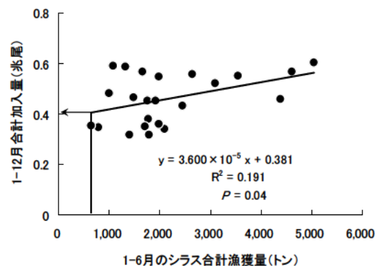
図18. シラス漁獲量と加入量の関係
