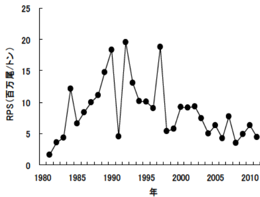
図11. RPSの経年推移
