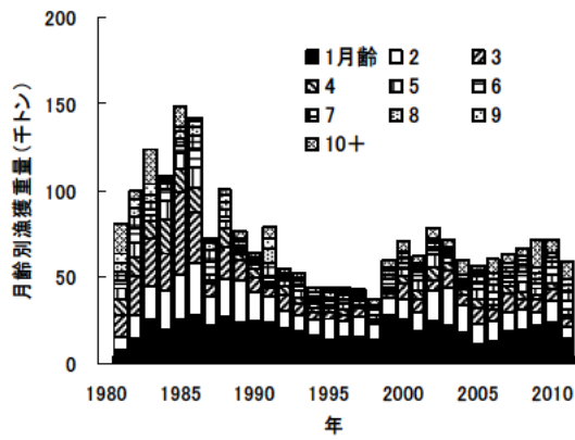
図7. 月齢別漁獲重量の経年推移
