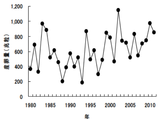
図6. 産卵量の経年推移
