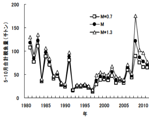
図13. Mの変化が親魚量に及ぼす影響
