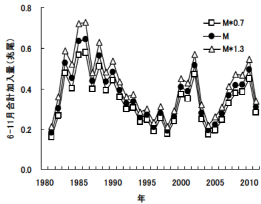
図14. Mの変化が加入量に及ぼす影響
