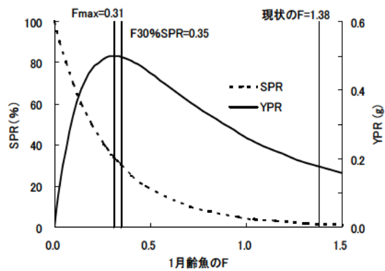
図19. YPRと%SPR
