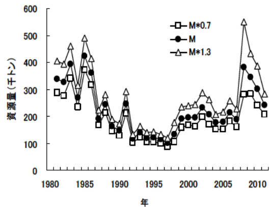
図12. Mの変化が資源量に及ぼす影響
