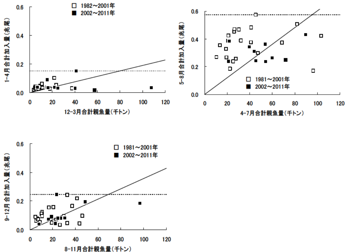
補足図 1. 3 半期別再生産関係 実線は過去 10 年間（2002～2011 年）の再生産成功率の中央値、点線は各 3 半期における加入量の上限值を示す。
