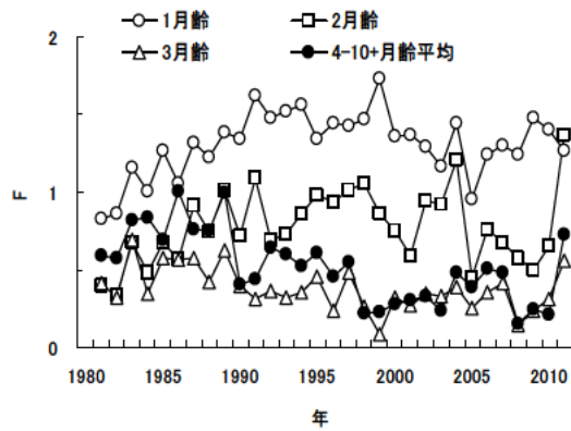
図15. Fの経年推移
