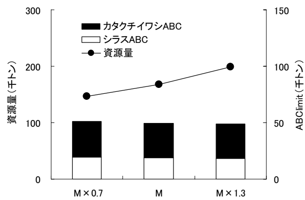
図25. Mを変化させた場合の2013年の資源量とABClimit
