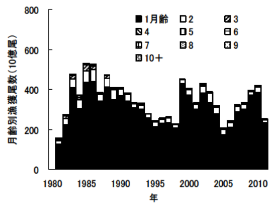
図8. 月齢別漁獲尾数の経年推移
