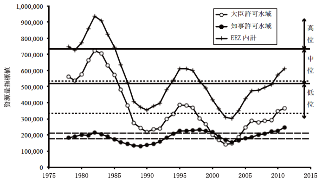
図6. 資源量指標値の経年変化
