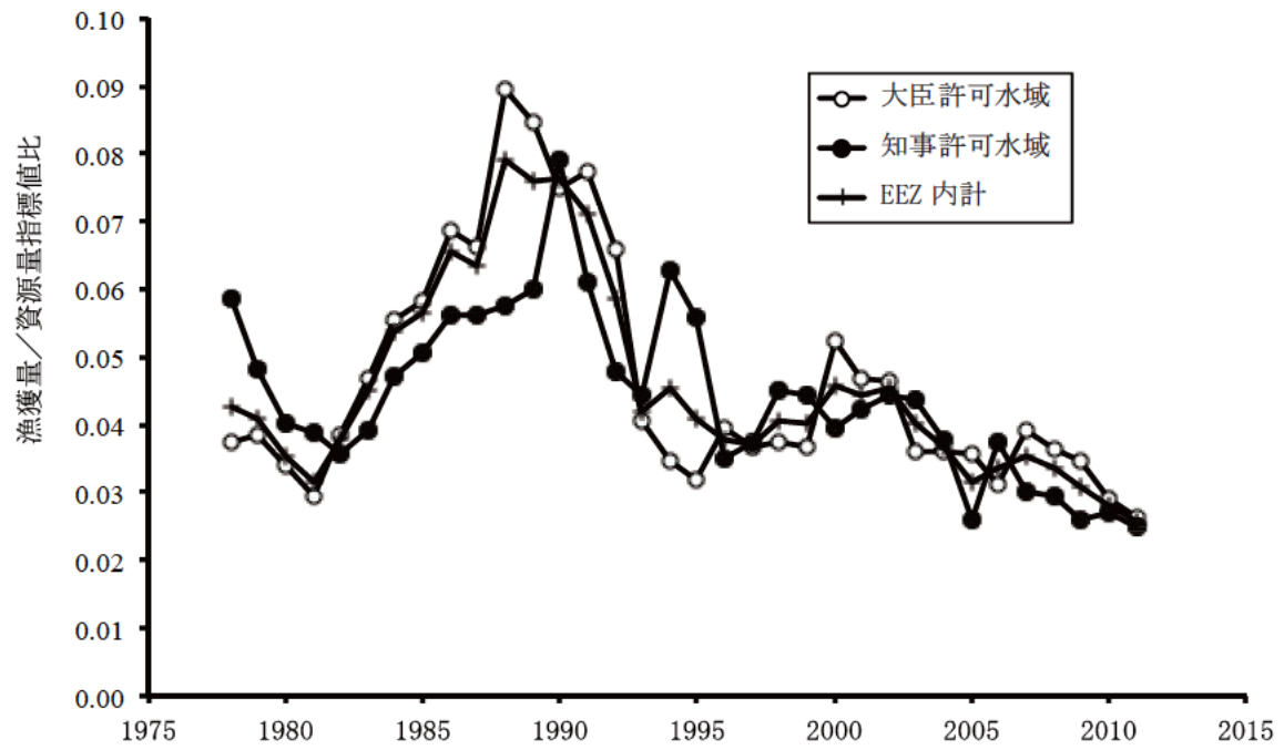
図7. 漁獲量/資源量指標値比の経年変化
