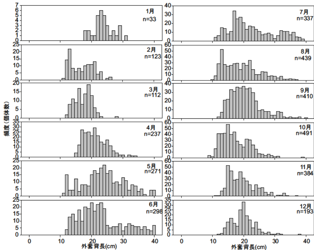
図 9. 沿岸いか釣り漁業によるケンサキイカ漁獲物体長組成 (2011 年)
