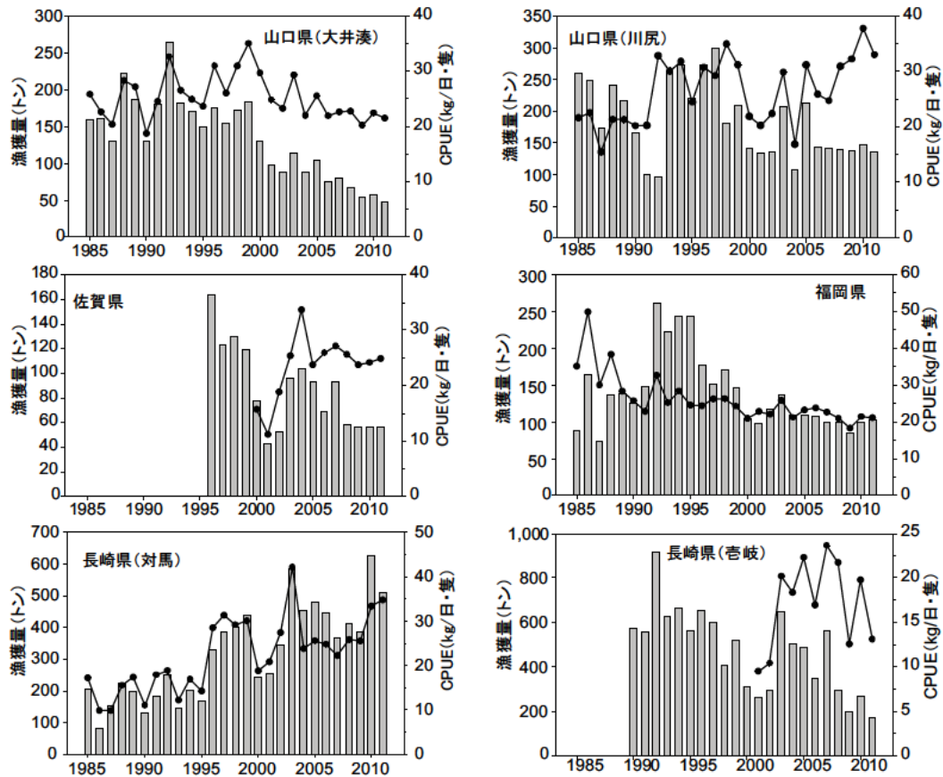
図 8. 各県代表港における沿岸いか釣り漁業による漁獲量と CPUE (漁獲量：棒グラフ、CPUE：折れ線グラフ)
