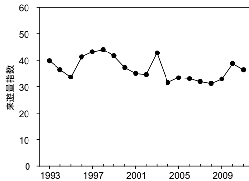
図 11. ケンサキイカ来遊量指数
