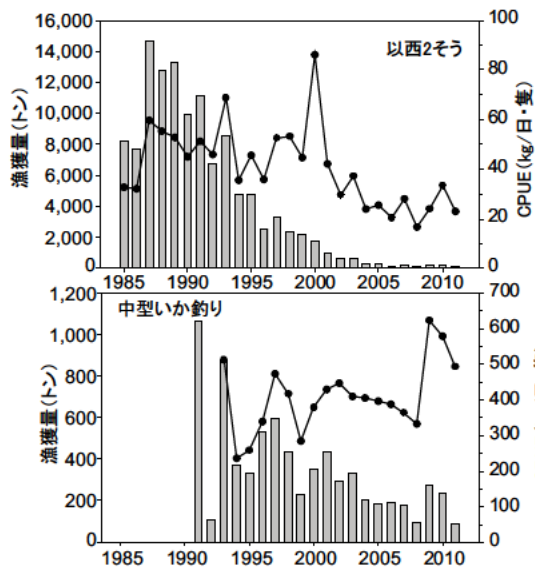
図 5. 海域別ケンサキイカ漁獲量
