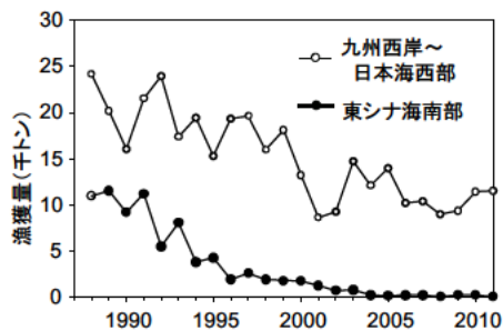
図 5. 海域別ケンサキイカ漁獲量
