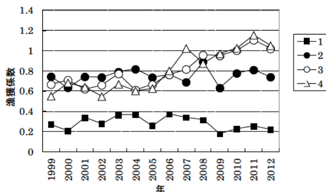
図 17. 年齢別の漁獲係数の推移
