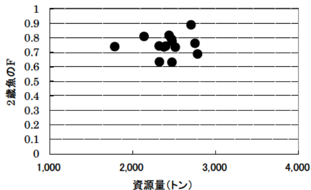
図 18. 資源量と 2 歳魚の漁獲係数(F)の関係
