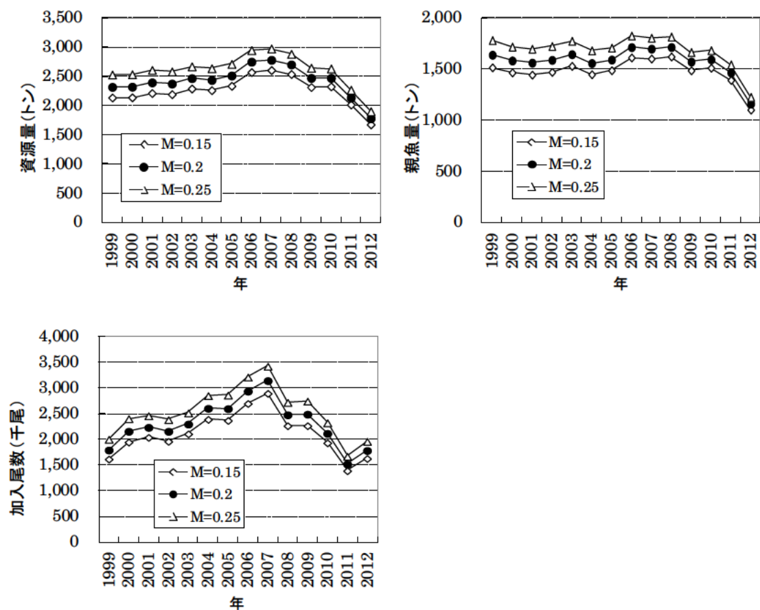
図 14. M を変化させたときの資源量 (左上)、親魚量 (右上)、加入尾数 (下) の変化
