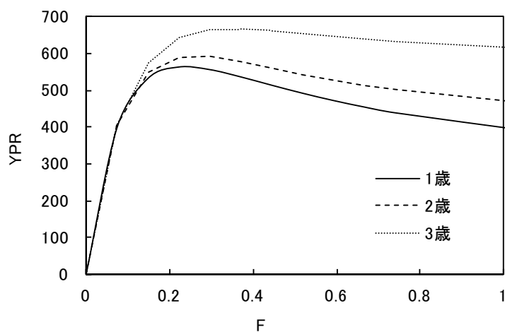
図 22. 漁獲開始年齢別の漁獲係数(F)と YPR の関係 現状は漁獲開始年齢 1 歳、 F=0.74 。
