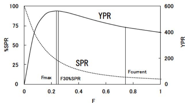
図 19. 2 歳魚の漁獲係数(F)と YPR、%SPR の関係
