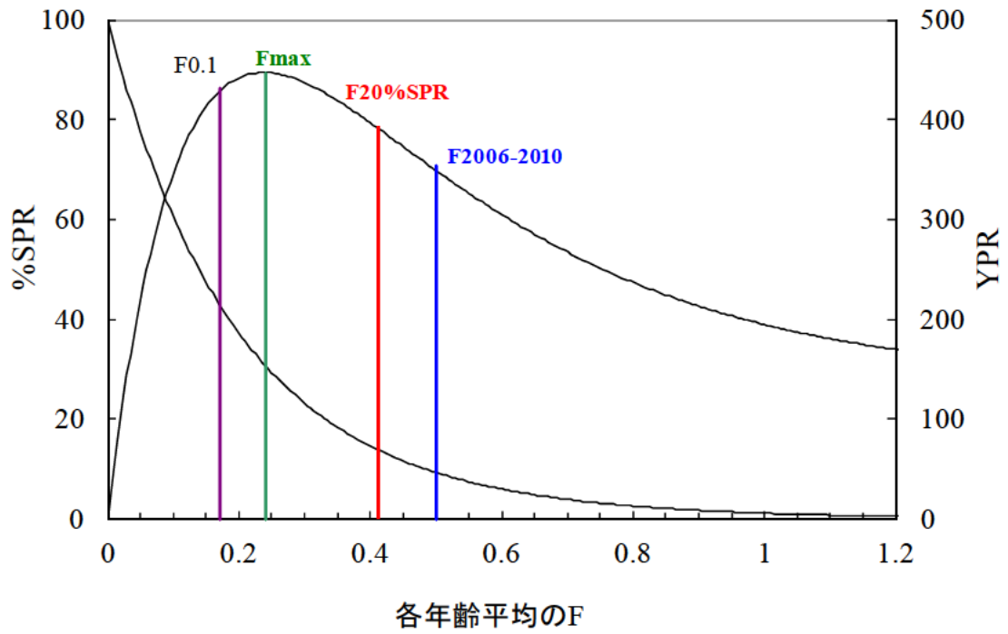
図 13. 漁獲係数、%SPR および YPR
