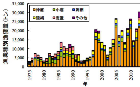
図 3. 太平洋北部におけるマダラの漁獲量 2013 年は暫定値。
