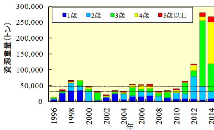
図 7. 年齢別資源量の経年変化 図中の破線は水準判断基準を示す。
