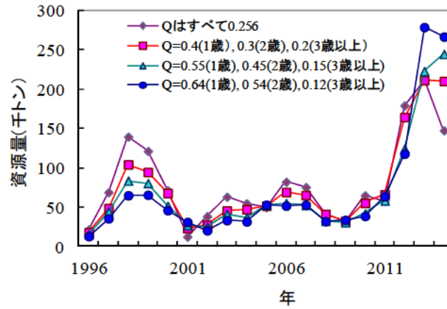
図 11. Q を変化させたときの資源量変化
