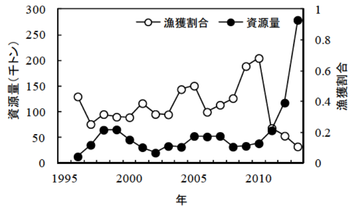
図 8. 資源量と漁獲割合の経年変化 2013 年の漁獲割合は暫定値。
