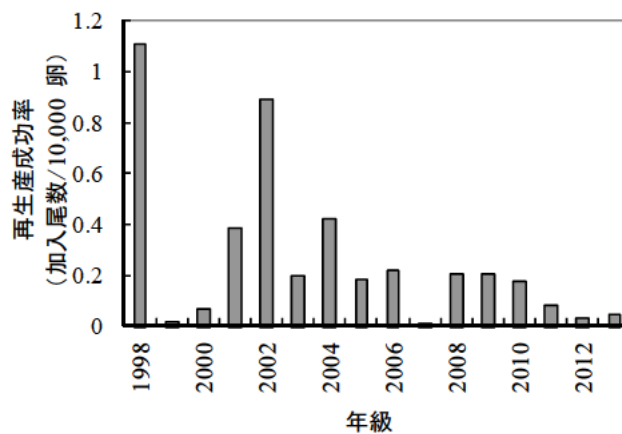
図 10. 再生産成功率の時系列変化
