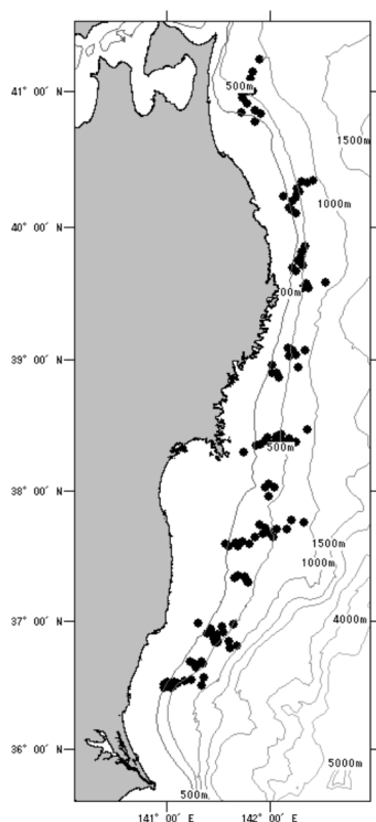
補足図 2. 2013 年 10～11 月の資源量調査点図
