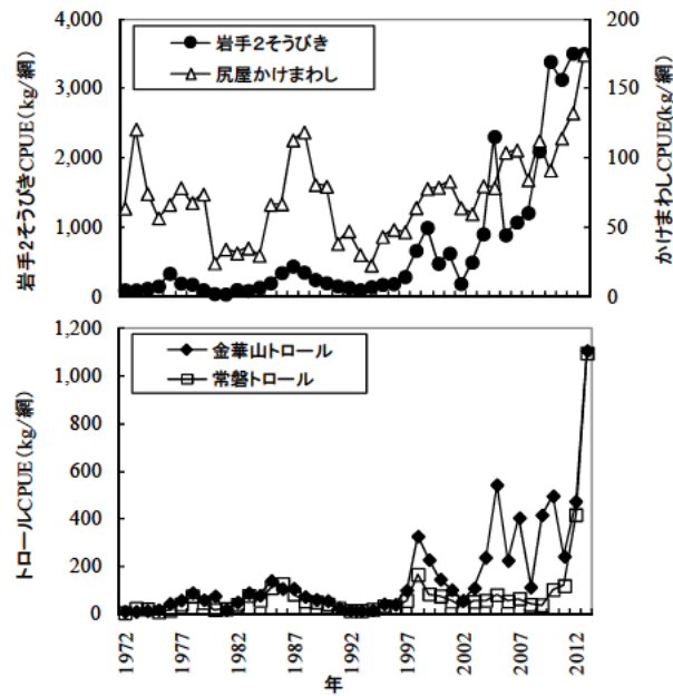
図 5. 沖底による CPUE の経年変化. 上：2 そうびきとかけまわし。 下：トロール. 2013 年は暫定値。
