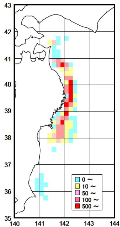
図 4. 沖底による 2012 年の漁獲量 (トン) の分布
