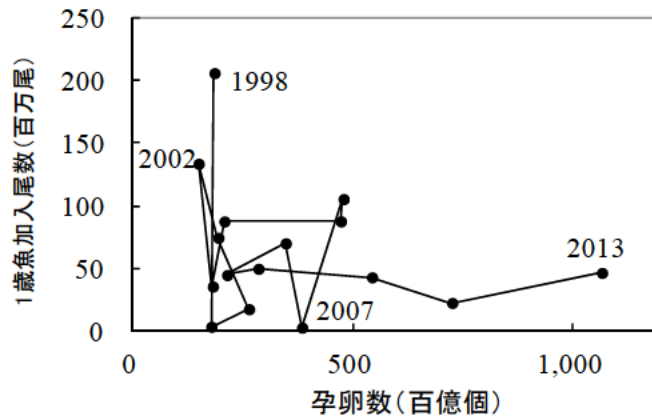
図 9. 再生産関係（孕卵数と加入尾数の関係） 数字は加入個体の年級。
