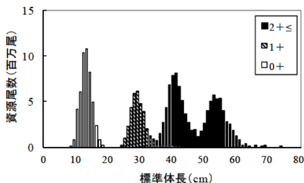
補足図 1. 調査におけるマダラの年齢別体長組成 年齢別採集効率は本文参照。
