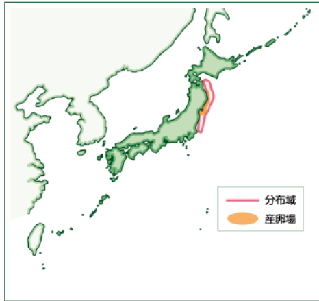
図 1. 太平洋北部におけるマダラ分布
