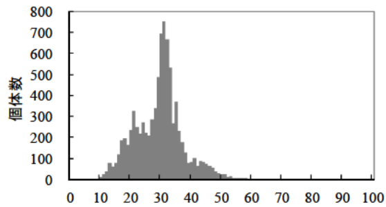
図 6. 2013 年に宮城県（石巻）に水揚げされたマダラの標準体長組成 (cm)。
