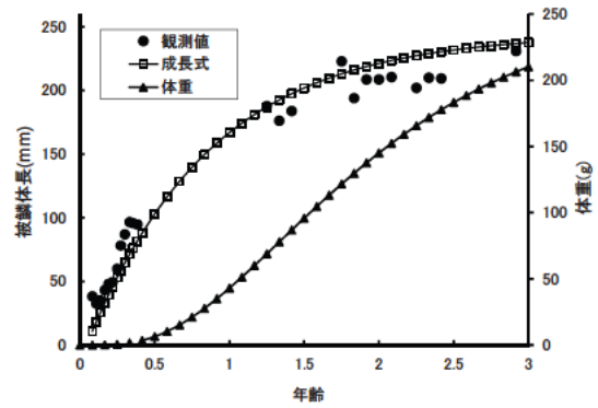
図 2. 月別体長組成から求めた成長式 ●は鱗と耳石日輪による年齢査定結果。
