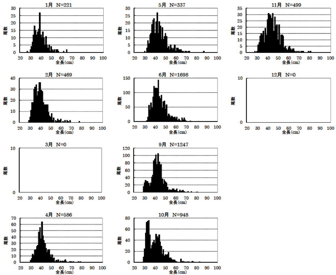
図 10. 新潟県岩船港における漁獲物の全長組成 (2014 年) 尾数は各月の調査尾数を示す。
