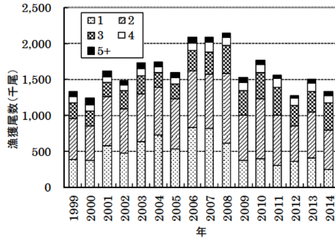
図 12. 年齢別漁獲尾数の推移 年齢起算日は1月1日。
