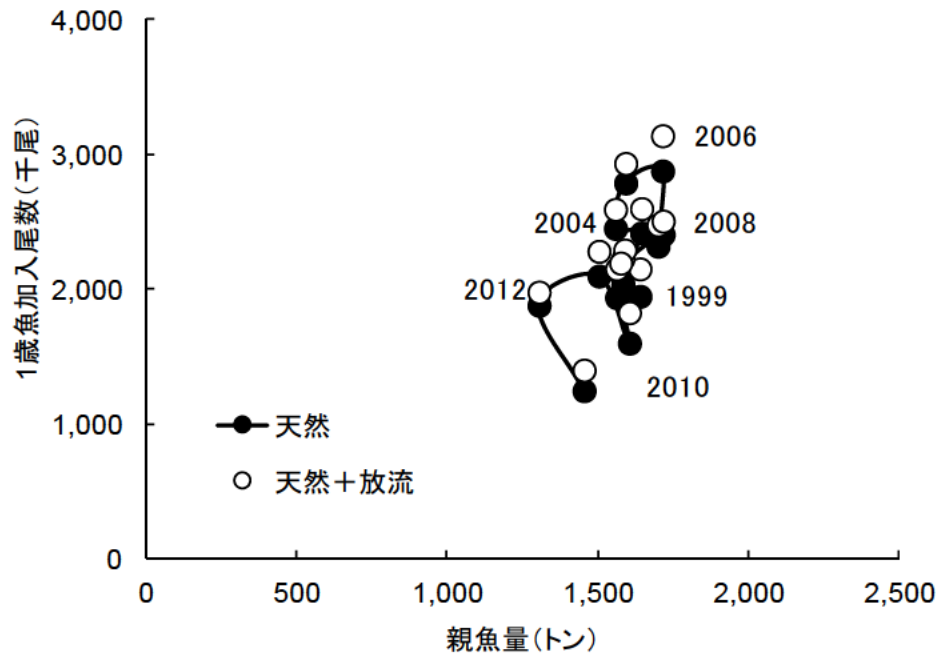
図 16. 前年の親魚量と 1 歳魚加入尾数
