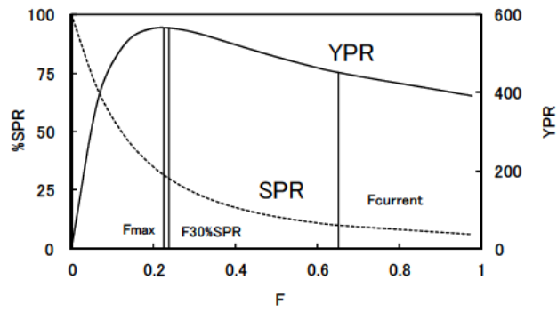
図 20. 2 歳魚の漁獲係数(F)と YPR、%SPR の関係
