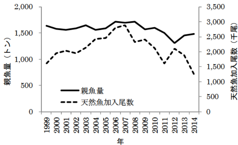
図 15. 親魚量と天然魚加入尾数の推移
