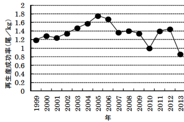
図 17. 再生産成功率の推移
