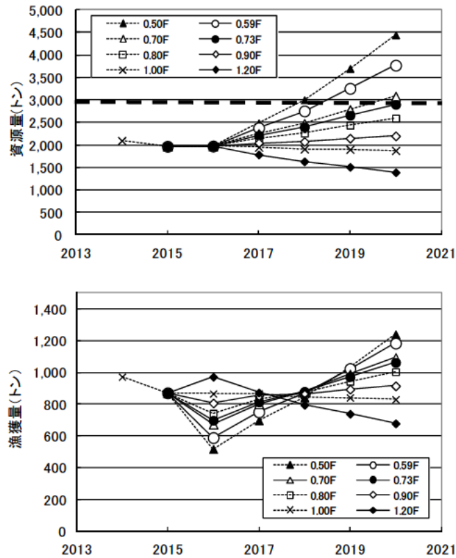
図 21. F の変化による資源量(上)と漁獲量(下)の推移 凡例内の F は F_{\text{current}}(0.65) 、数値は F_{\text{current}} に対する係数。 0.73F = F_{\text{rec}} 、 0.59F = 0.8 \times F_{\text{rec}} 。 資源量(上)に示した横鎖線は B_{\text{limit}} (2,900 トン)。
