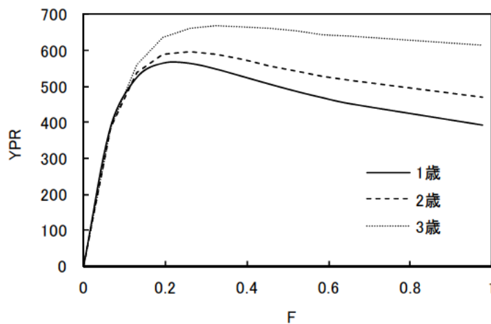
図 22. 漁獲開始年齢別の漁獲係数(F)と YPR の関係 現状は漁獲開始年齢 1 歳、 F = 0.65 。
