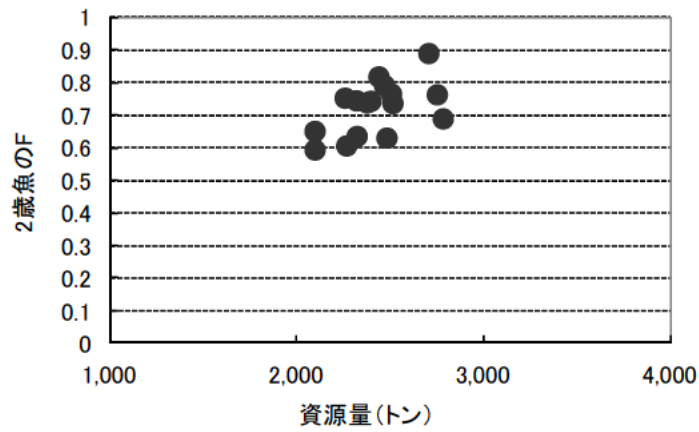
図 19. 資源量と 2 歳魚の漁獲係数(F)の関係
