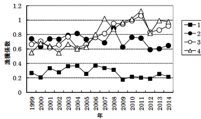
図 18. 年齢別の漁獲係数の推移
