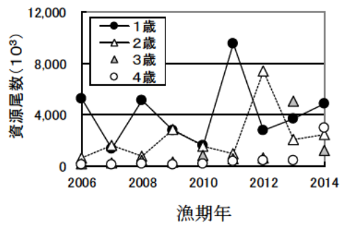
図 10. 年齢別資源尾数（全域）
