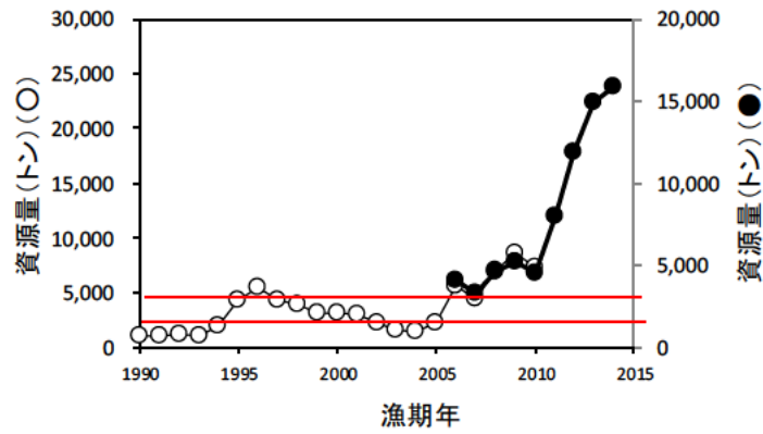
図 8. 1990～2014 年漁期年資源量の推移（全域）
