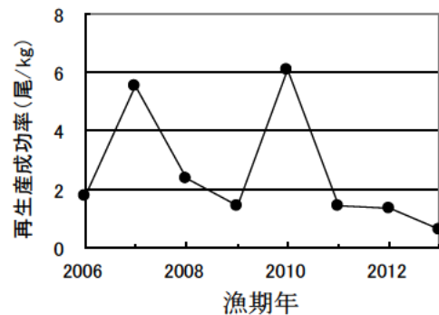
図 18. 再生産成功率の推移 再生産成功率は翌年 1 歳加入尾数を当年の雌の SSB で除して求めた。
