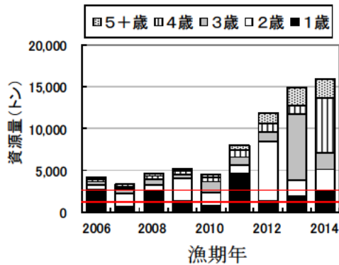
図 9. 年齢別資源量（全域）
