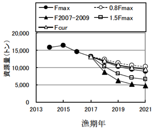
図 20. F を変化させた時の資源量の変化 (全域)
