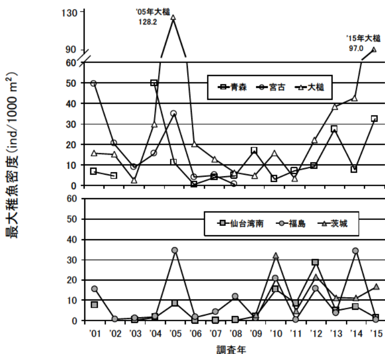
補足図5-1. 東北北部海域(上)と南部海域(下)におけるヒラメ着底稚魚密度の経年変化
