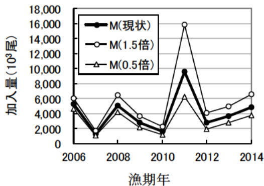
図 17. M の感度解析（加入量）
