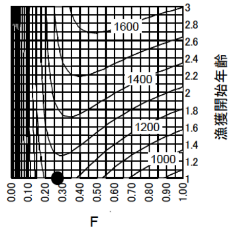
図 22. F および漁獲開始年齢を変化させた時の太平洋北部系群の加入あたり漁獲量の変化 雌の値のみを用いて作図した。黒丸は 2014 漁期年の値を表す。図中の数字は g。
