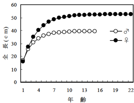
図3. サメガレイの成長
