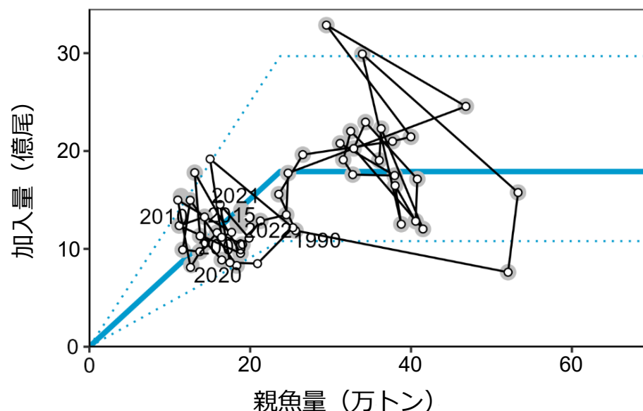
図6 再生産関係
