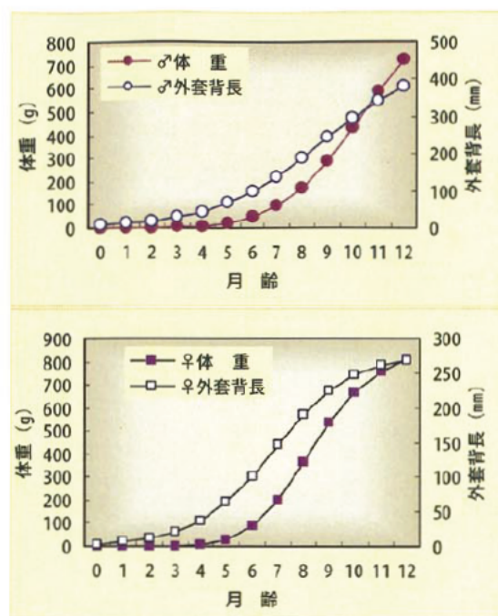
図2 ケンサキイカ年齢・成長関係
