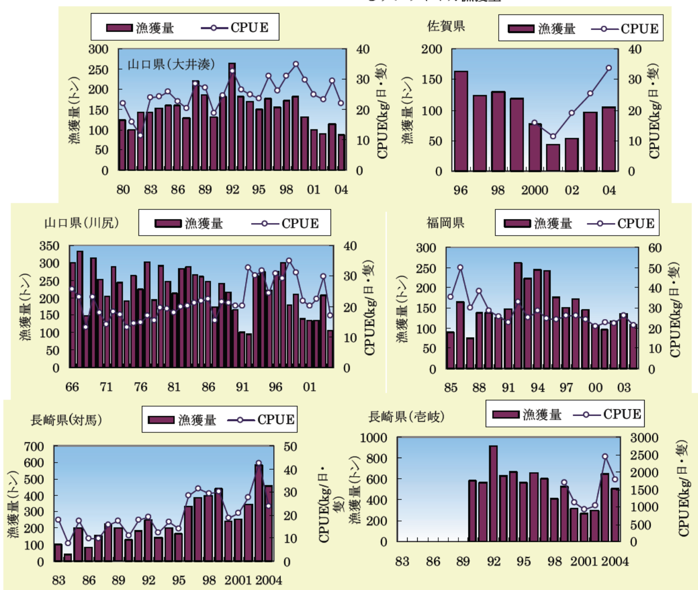
図7 各県代表港における沿岸イカ釣り漁業による漁獲量と CPUE
