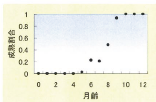
図3 ケンサキイカ年齢別成熟割合図
