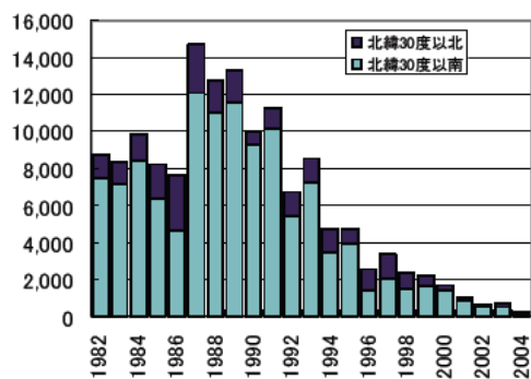
図6 海域別の以西底びき網漁業によるケンサキイカ漁獲量
