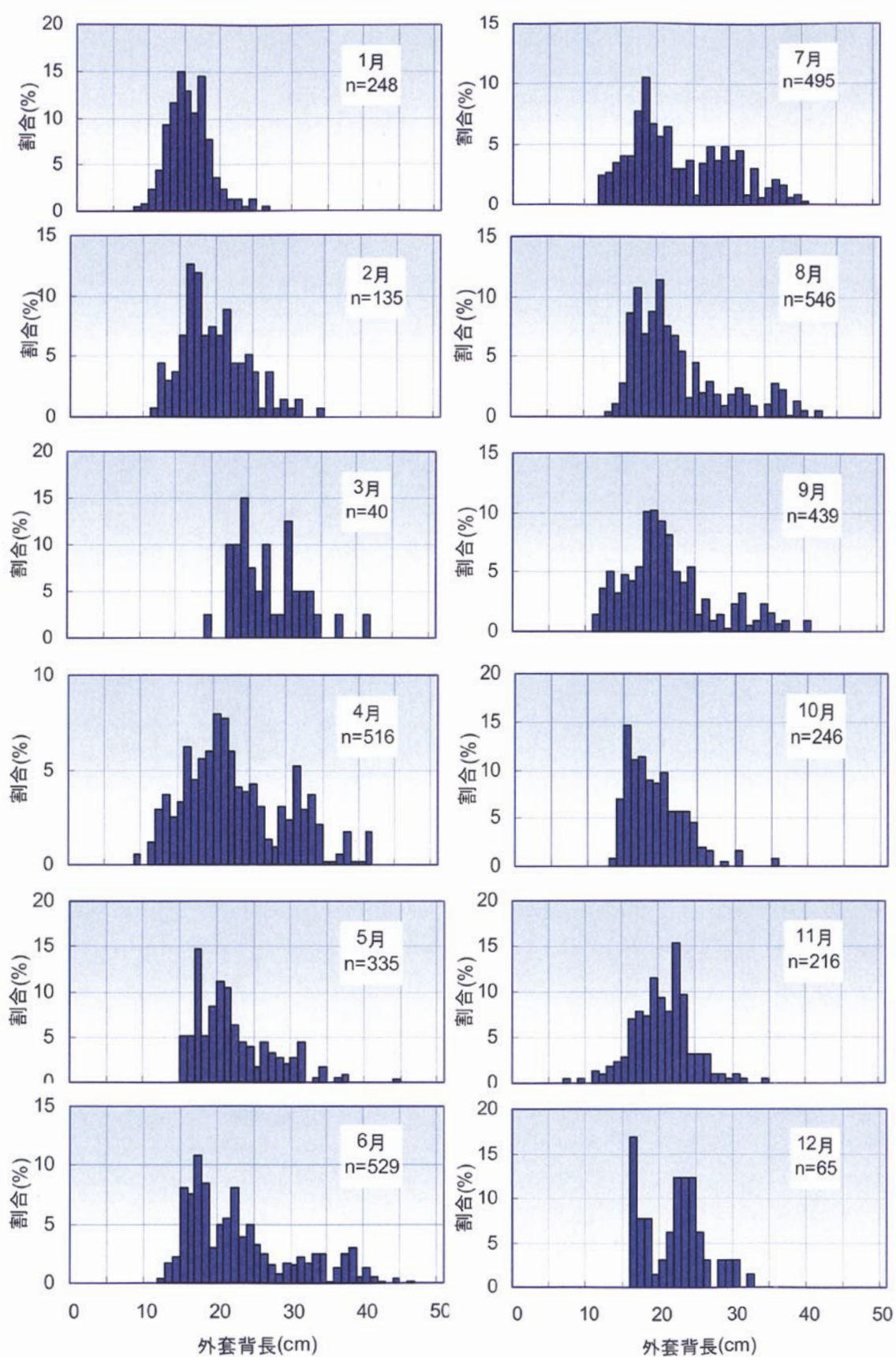
図 10 沿岸イカ釣り漁業によるケンサキイカ漁獲物体長組成
