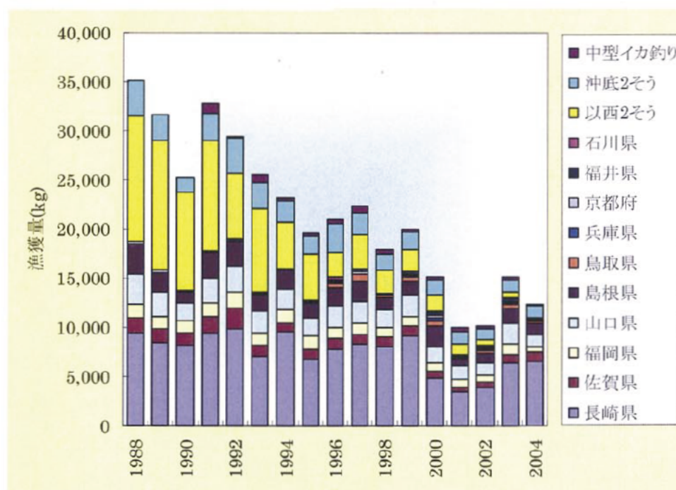
図4 ケンサキイカ漁獲量の経年変化
