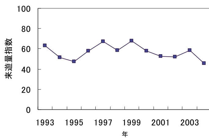
図 12 ケンサキイカ来遊量指数
