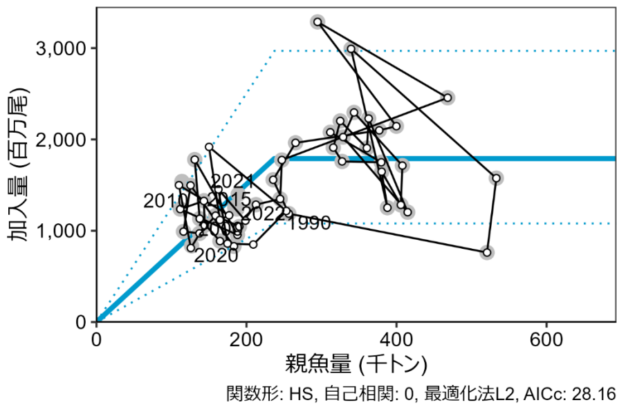
図 4-11. 親魚量と加入量の関係 (再生産関係) 平成 31 年 4 月に開催された「管理基準値等に関する研究機関会議」(安田ほか 2019) で提案された再生産関係式と再生産関係のプロット (灰色の丸印)。図中の再生産関係式 (青実線) の上下の点線は、仮定されている再生産関係において観察データの 90%が含まれると推定される範囲である。実線と白抜き丸印で示したのは今年度の評価で得られた再生産関係のプロット。図中の数字は年級群を示す。
