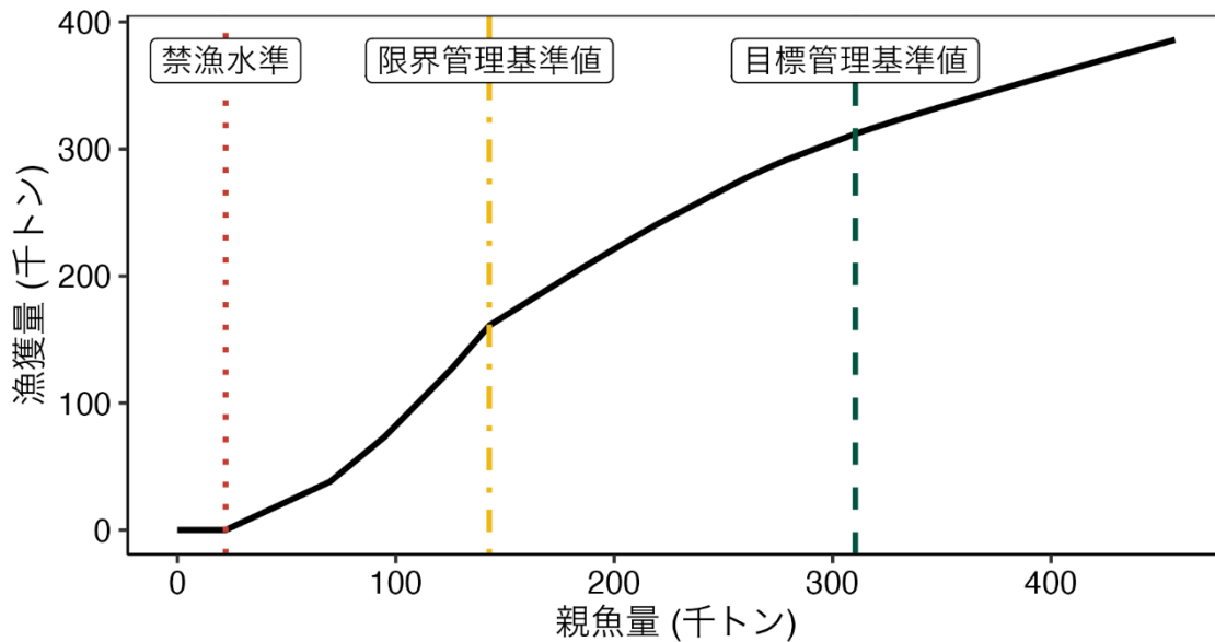
図 5-1. 漁獲管理規則（調整係数 \beta=0.95 の場合） 目標管理基準値（SBtarget）はホッケ-スティック型再生産関係に基づき算出した SB_{msy} である。限界管理基準値（ SB_{limit} ）および禁漁水準（ SB_{ban} ）にそれぞれ標準値を用いている。黒破線： F_{msy} 、灰色破線： 0.95F_{msy} 、黒太線： HCR 、赤点線：禁漁水準、黄色一点鎖線：限界管理基準値、緑色破線：目標管理基準値を示す。a) は縦軸を漁獲圧にした場合、b) は縦軸を漁獲量で表した場合である。b) については、漁獲する年の年齢組成によって漁獲量は若干異なるが、ここでは平衡状態における平均的な年齢組成の場合の漁獲量を示した。
