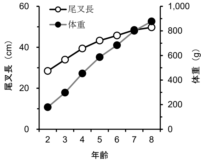
図 2-3. 沖底漁獲物の年齢別平均尾叉長と平均体重 (2013~2022 年の 4~7 月)
