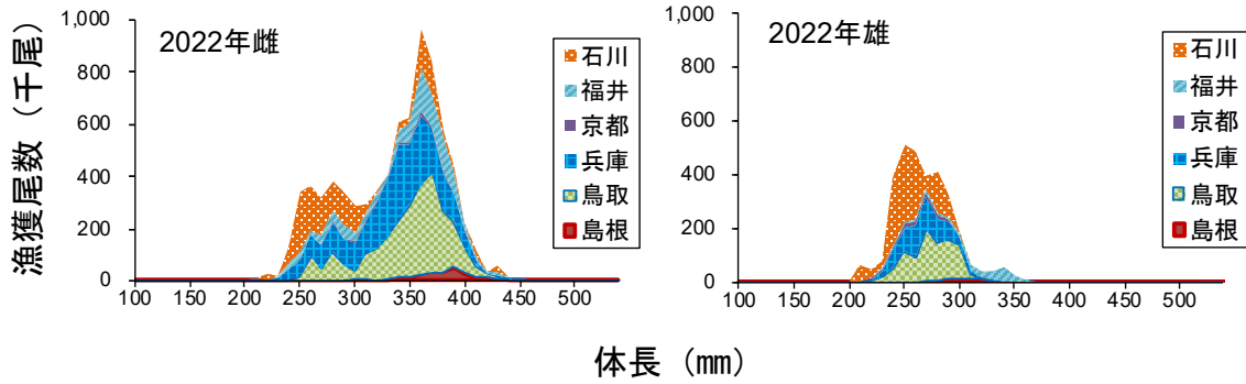
補足図 8-2. 日本海西部におけるアカガレイの漁獲物の雌雄別および府県別の体長組成
