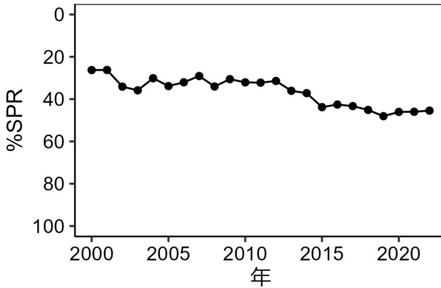
図 4-5. %SPR の推移 %SPR は漁獲がないときの親魚量に対する漁獲があるときの親魚量の割合を示し、F が高い（低い）と%SPR は小さく（大きく）なる。
