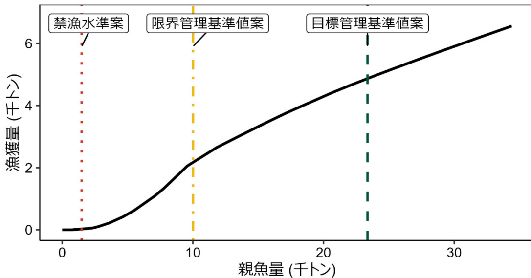
補足図 4-1. 漁獲管理規則案 目標管理基準値 (SBtarget) 案は HS 型再生産関係に基づき算出した SB_{msy} である。限界管理基準値 (SBlimit) 案および禁漁水準 (SBban) 案には、それぞれ標準値を用いている。調整係数 \beta には標準値である 0.8 を用いた。黒破線は F_{msy} 、灰色破線は 0.8F_{msy} 、黒太線は HCR、赤点線は禁漁水準案、黄一点鎖線は限界管理基準値案、緑破線は目標管理基準値案を示す。a) は縦軸を漁獲圧にした場合、b) は縦軸を漁獲量で表した場合である。b) については、漁獲する年の年齢組成によって漁獲量は若干異なるが、ここでは平衡状態における平均的な年齢組成の場合の漁獲量を示した。
