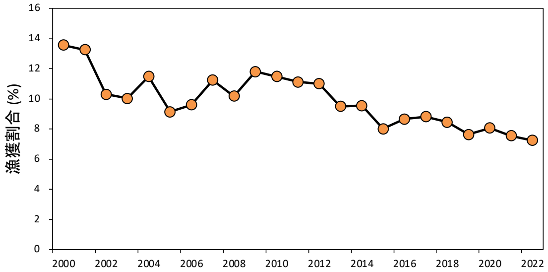
図 4-4. 漁獲割合の推移
