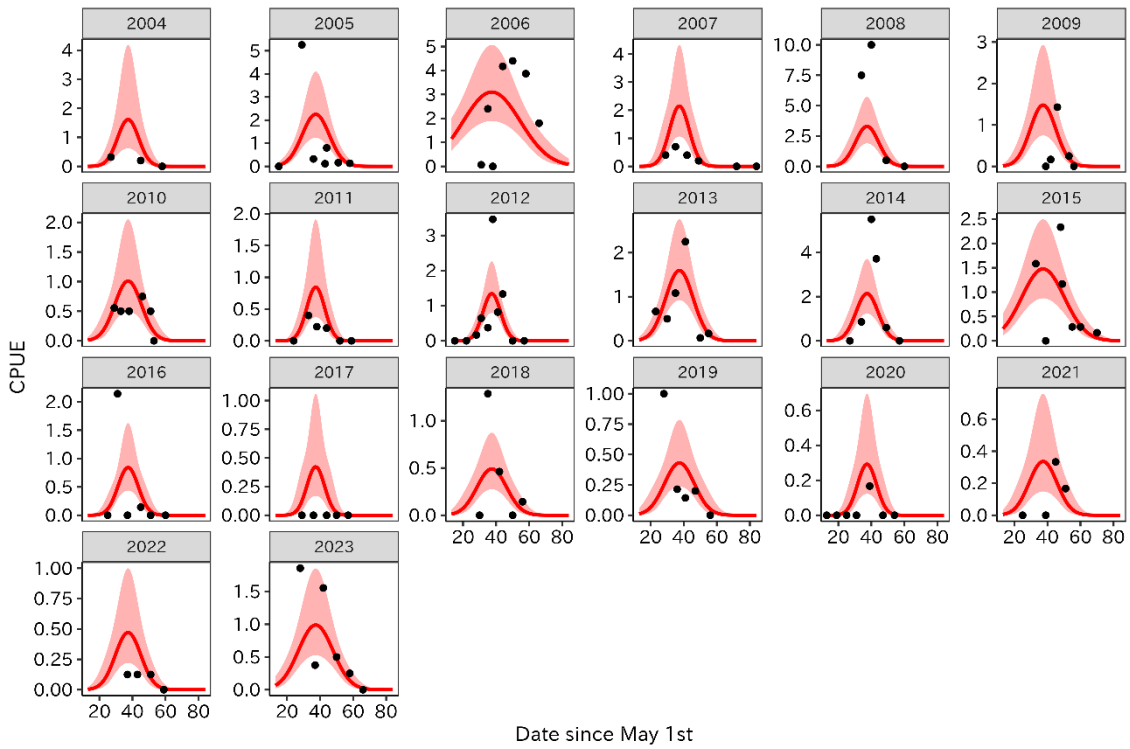
補足図 3-8. CPUE の観測値 (黒点) と予測値 (赤線) の漁期年別の経日推移 (横軸は 5 月 1 日からの日数) 赤い影は 80%信頼区間を表す。縦軸スケールが漁期年によって変わる点に注意。
