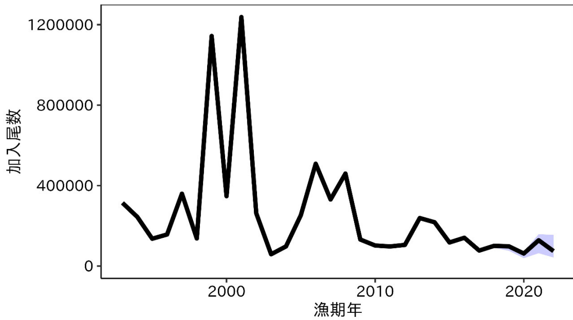
補足図 2-11. 加入量のノンパラメトリックブートストラップ解析結果 紫の影は 90%信頼区間を示す。
