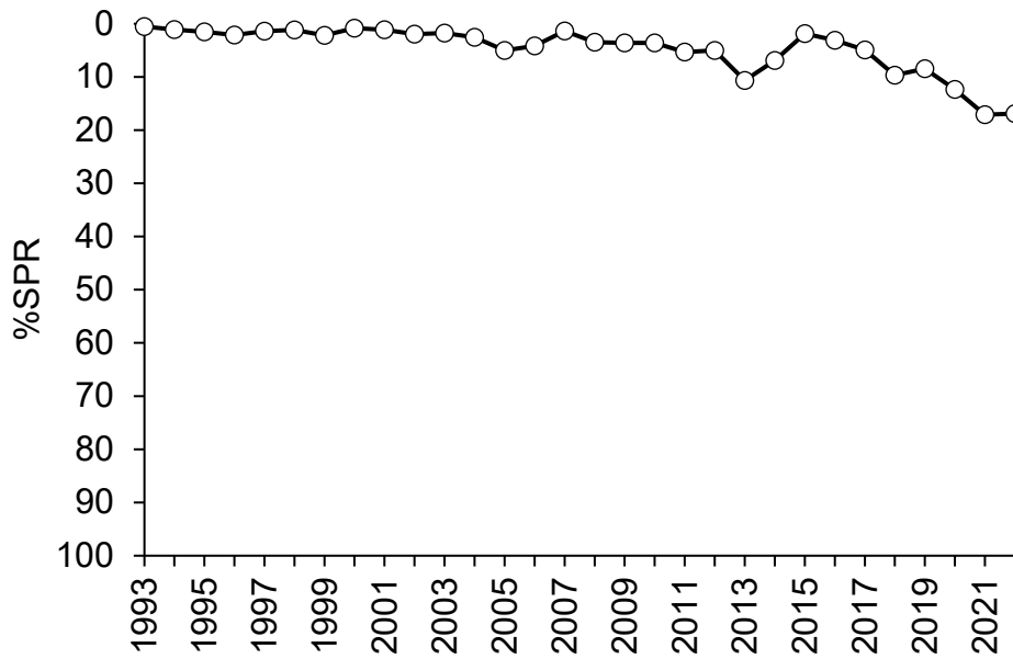
図 4-12. 各漁期年における%SPR 値の経年推移
