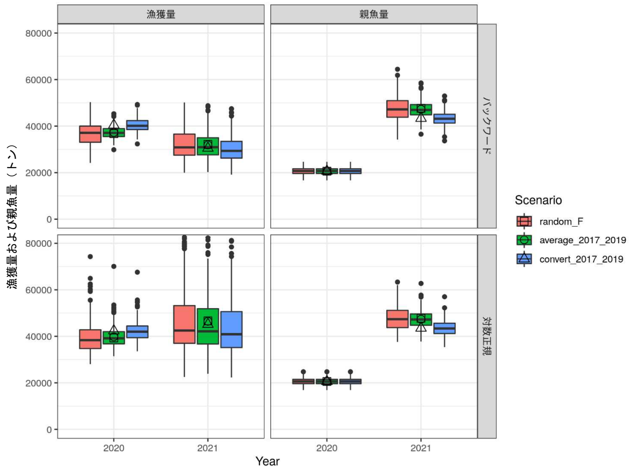
補足図 3-1. 2020 年の漁獲圧 ( F 値) の仮定の違いによる 2020 年および 2021 年の漁獲量 (左) と親魚量 (右) の比較 (シミュレーション回数は 300 回)。上はバックワート・リサンプリングの加入を仮定した場合 (ホッケー・スティック型再生産関係を用いた低加入シナリオによる予測)、下は通常の対数正規分布を仮定した場合 (ホッケー・スティック型再生産関係を用いた通常加入の予測)。中央に示された白抜きのシンボルはそれぞれ凡例の場合の平均値。
