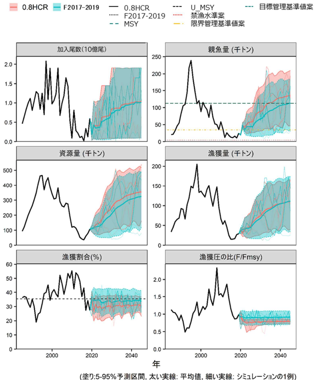
補足図 2-2. 漁獲管理規則案を用いた場合と現状の漁獲圧（F2017-2019）で漁獲を続けた場合とでの将来予測の比較
