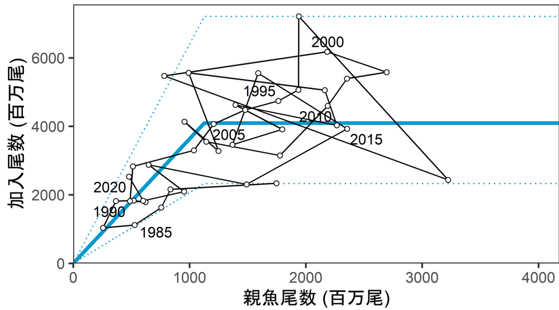
図 2. 親魚量と加入量の関係（再生産関係） 青線は令和 2 年 7 月に開催された「管理基準値等に関する研究機関会議」において適用された再生産関係式 青実線は再生産関係を、上下の青点線は仮定されている再生産関係において観察データの 90%が含まれると推定される範囲である。黒線は本資源評価で新たに推定された加入尾数、親魚尾数のプロットで、図中の推移時は年級群を示す。2020 年漁期の親魚尾数は F2020（予測値）による漁獲後の残存資源尾数の推定値。
