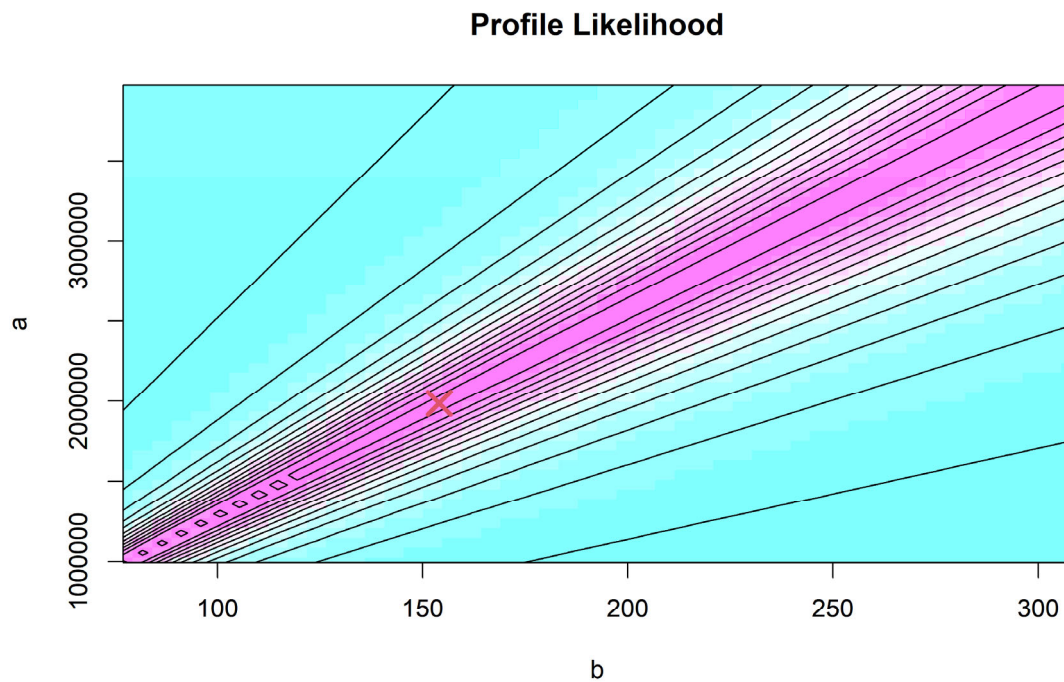
補足図 1-8b. ベバートン・ホルト型再生産関係式を最小二乗法で当てはめた場合の推定パラメータのプロファイル尤度
