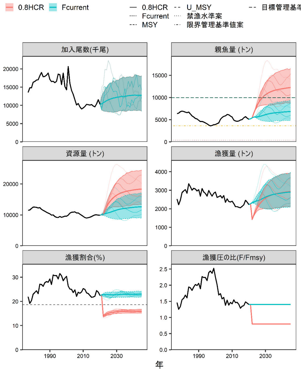
補足図 2-5. 再生産関係に自己相関を考慮したホッケー・スティック (HS) 型再生産関係式を用いた場合の、管理基準値案に基づく漁獲管理規則案を用いた将来予測 (赤色) と現状の漁獲圧で漁獲を続けた場合の将来予測 (緑色) の比較 太実線は平均値、網掛けはシミュレーション結果の 90%が含まれる 90%予測区間、細線は 3 通りの将来予測の例示である。親魚量の図の緑破線は目標管理基準値案、黄破線は限界管理基準値案、赤線は禁漁水準案を示す。漁獲割合の図の破線は U msy を示す。2021 年の漁獲は予測される資源量と現状の漁獲圧 (F current ) により仮定し、2022 年以降の漁獲は漁獲管理規則案 (補足図 2-4) に従うものとした。調整係数 \beta には 0.8 を用いた。
