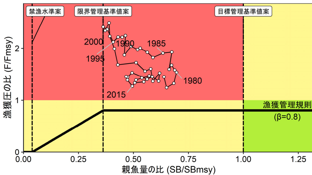
補足図 2-3. 再生産関係に自己相関を考慮したホッケ－・スティック (HS) 型再生産関係式を用いた場合の神戸プロット
