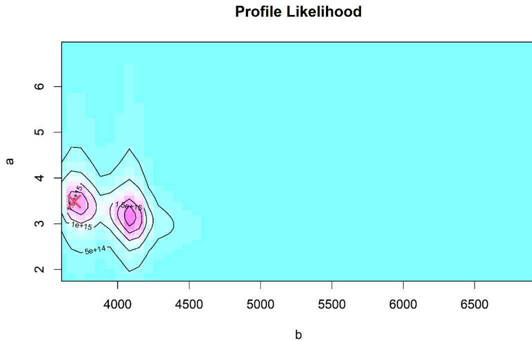
補足図 1-8a. ホッカー・スティック型再生産関係式を最小二乗法で当てはめた場合の推定パラメータのプロファイル尤度
