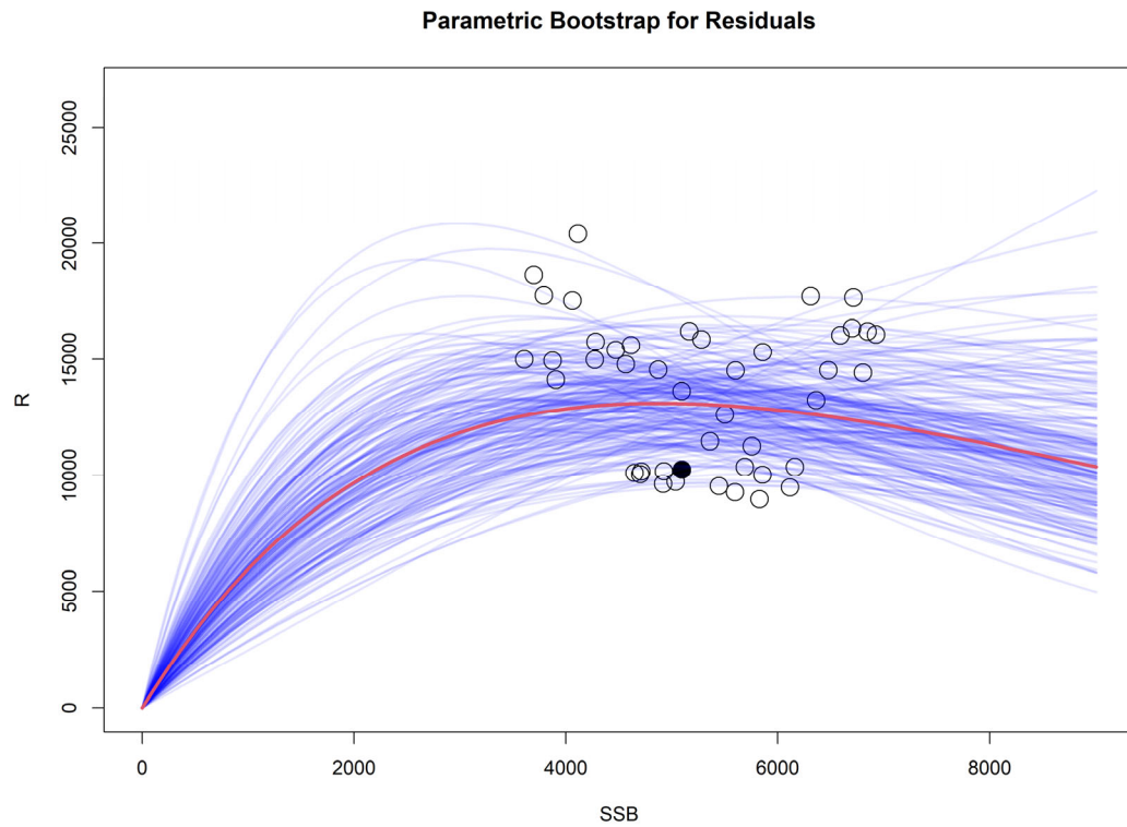
補足図 1-6c. リッカー型再生産関係式を最小二乗法で当てはめた場合の残差ブートストラップ解析の結果
