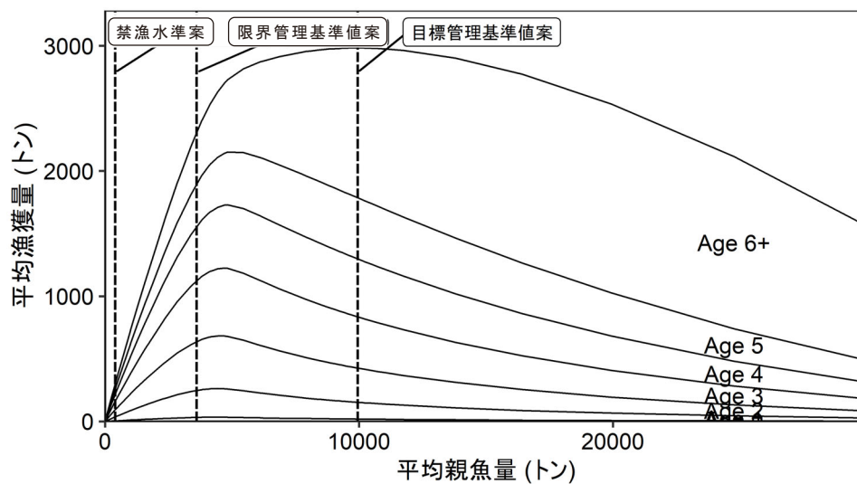
補足図 2-2. 再生産関係に自己相関を考慮したホッケ－・スティック（HS）型再生産関係式を用いた場合の管理基準値案および禁漁水準案と年齢別漁獲量曲線の関係
