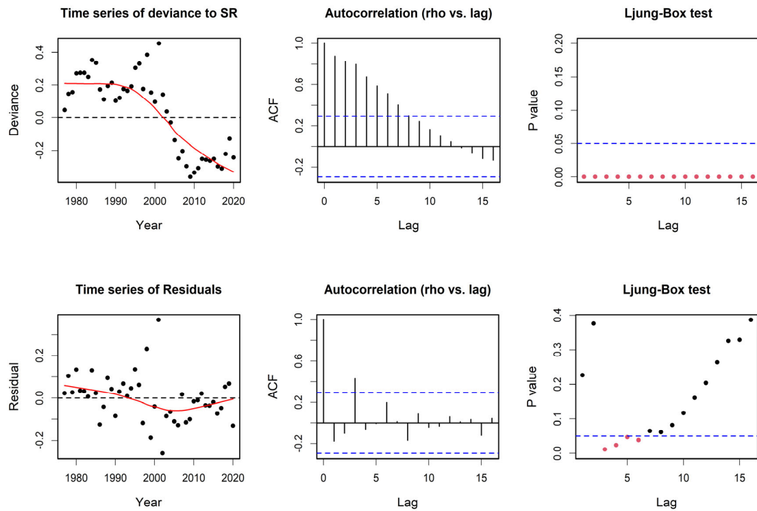
補足図 1-2c. リッカー型再生産関係式を最小二乗法で当てはめた場合の、再生産関係との逸脱度 (deviance) および自己相関を同時推定で考慮した残差 (residual) のトレンド (左図)、自己相関プロット (中央図)、および Ljung-Box 検定における P 値 (右図) 残差の時系列の図中の赤線は平滑化された曲線を示す。自己相関プロットの青色の点線は 95%信頼区間を示す。Ljung-Box 検定における P 値 (縦軸) の青色の点線は 5%水準を表す。
