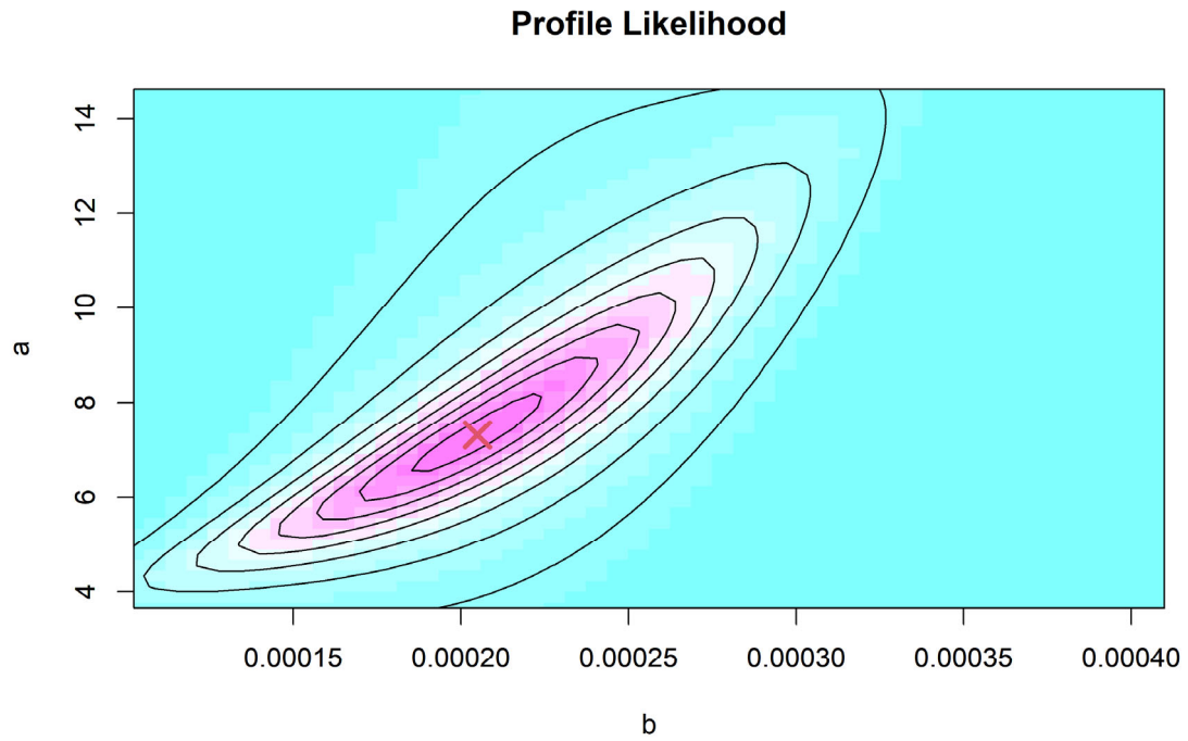
補足図 1-8c. リッカー型再生産関係式を最小二乗法で当てはめた場合の推定パラメータのプロファイル尤度 ×印は推定されたパラメータ値における尤度に相当する。
