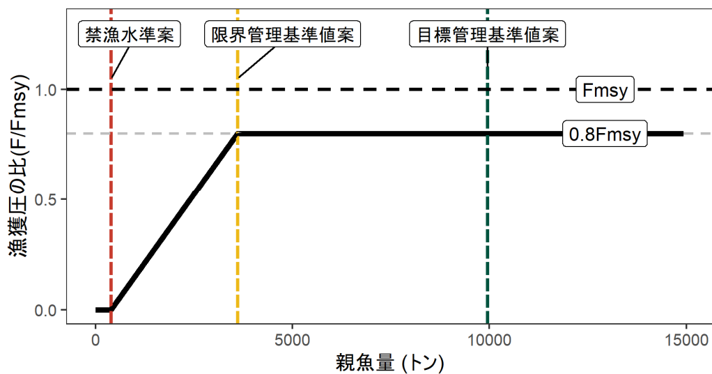
補足図 2-4. 再生産関係に自己相関を考慮したホッケ－・スティック (HS) 型再生産関係式を用いた場合の漁獲管理規則 (HCR) 案
