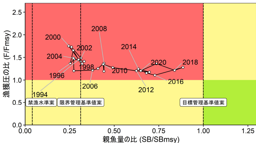
図4. 神戸プロット
