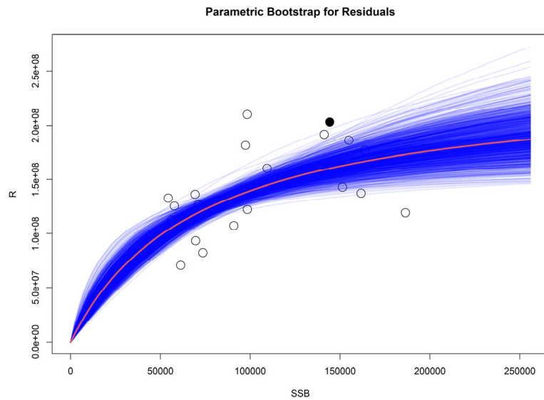
補足図 1-6b. BH 型再生産関係式を最小二乗法で当てはめた場合の残差ブートストラップ解析の結果
