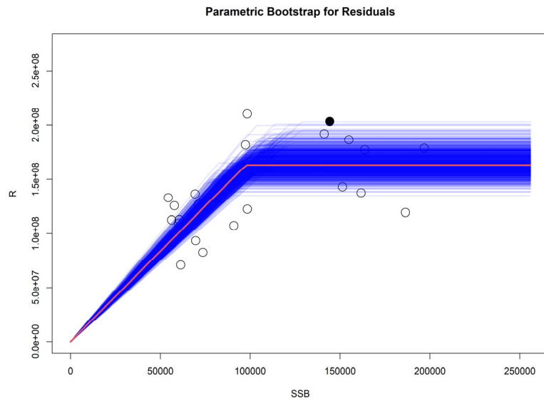
補足図 1-6a. HS 型再生産関係式を最小二乗法で当てはめた場合の残差ブートストラップ解析の結果
