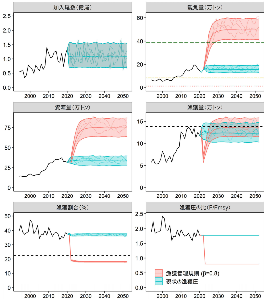
補足図 4-4. 管理基準値案に基づく漁獲管理規則案を用いた将来予測（赤色）と現状の漁獲圧で漁獲を続けた場合の将来予測（緑色）の比較
