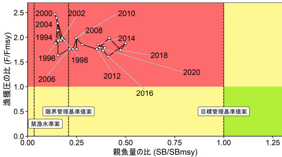
補足図 8-2. 神戸プロット
