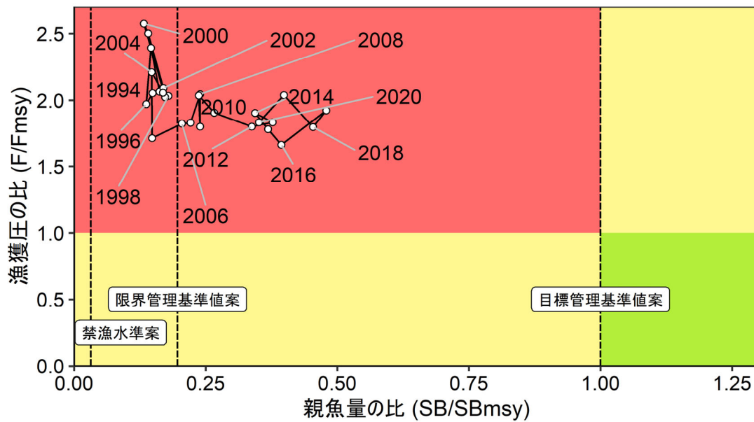
補足図 7-2. 神戸プロット
