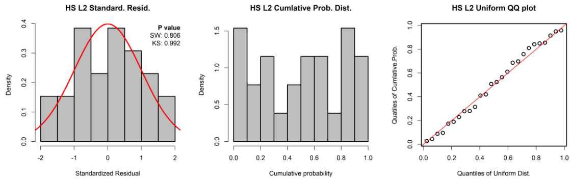
補足図 1-5. 最小二乗法により推定した自己相関を考慮した HS 型再生産関係の残差分布の正規性の検定結果と QQ プロット
