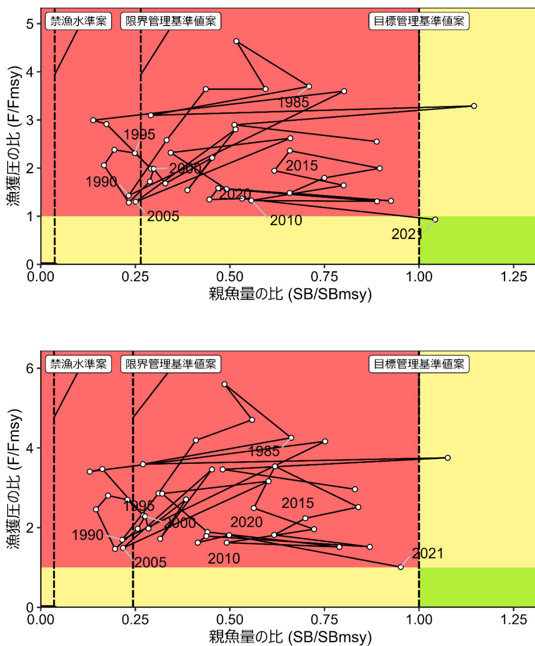
補足図 4-3. 神戸プロット
