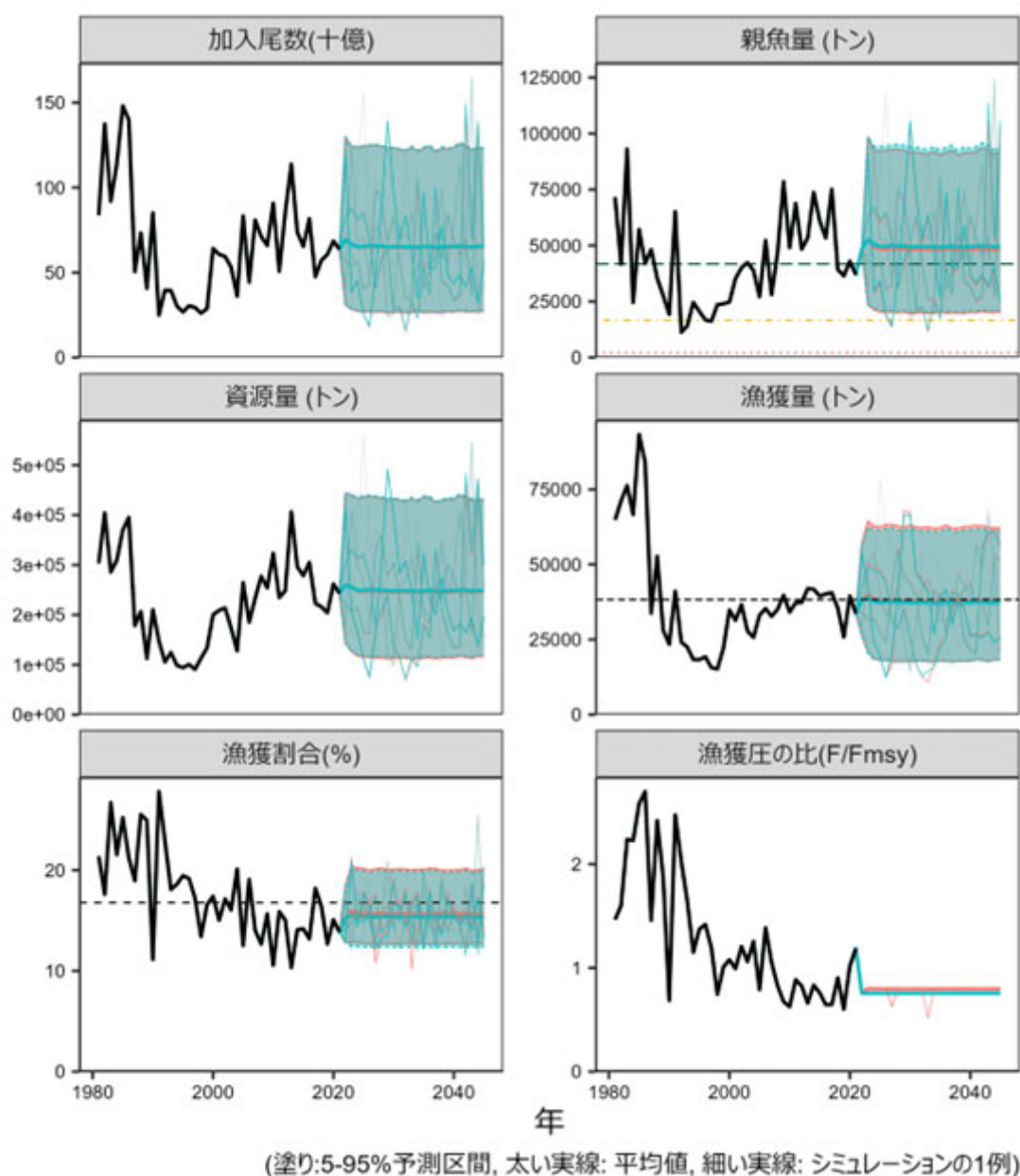
補足図 3-6. 管理基準値案に基づく漁獲管理規則案を用いた将来予測（赤色）と現状の漁獲圧で漁獲を続けた場合の将来予測（緑色）の比較
