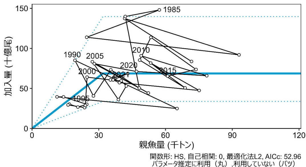
補足図 3-1. 再生産関係
