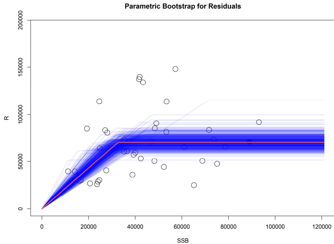
補足図 1-6. ホッケー・スティック型再生産関係式を最小二乗法で当てはめた場合の残差ブートストラップ解析の結果 赤線は元データでの推定値、青線はパラメトリックブートストラップでの推定値である。横軸は親魚量（トン）、縦軸は加入尾数（百万尾）である。丸印は分析に使用した親魚量・加入尾数であり、黒丸は使用していない 2021 年を示す。
