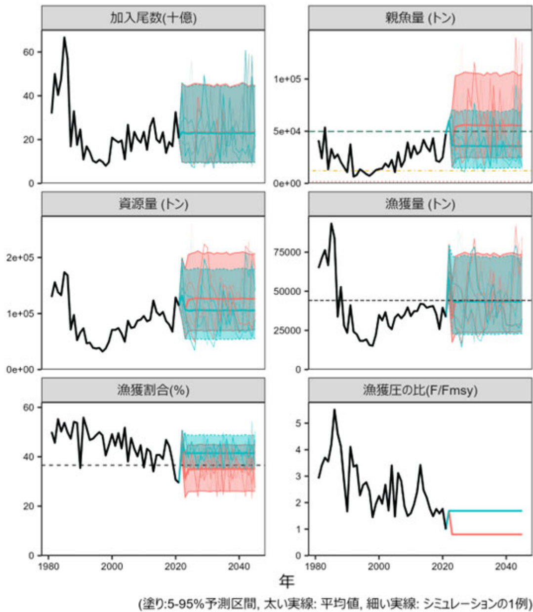
補足図 4-7. 管理基準値案に基づく漁獲管理規則案を用いた将来予測（赤色）と現状の漁獲圧で漁獲を続けた場合の将来予測（緑色）の比較 対馬暖流系群の M を適用した場合である。
