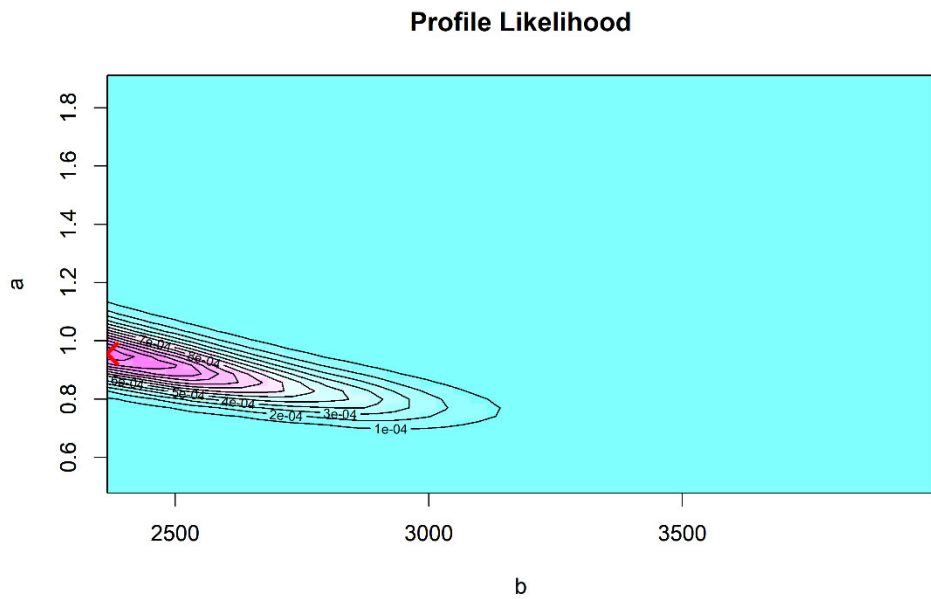
補足図 1-8a. 自己相関を考慮したホッケー・スティック型 (HS) 再生産関係式を最小二乗法で当てはめた場合の推定パラメータのプロファイル尤度 ×印は推定されたパラメータ値における尤度に相当する。
