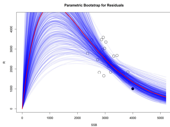
補足図 1-6b. リッカー型再生産関係式を最小二乗法で当てはめた場合の残差ブートストラップ解析の結果
