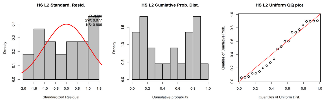
補足図 1-3a. ホッケー・スティック型再生産関係式を最小二乗法で当てはめた場合の標準化残差のヒストグラムと正規性テスト結果（左図）、残差の累積確率密度のヒストグラム（中央図）、および一様分布を仮定した QQ プロット（右図） 残差のヒストグラムの右上の数値は Shapiro-Wilk 検定（SW）と Kolmogorov-Smirnov 検定（KS）の結果である。どちらも、帰無仮説は「正規分布に従っている」である。QQ プロットの赤線は理論値を示している。
