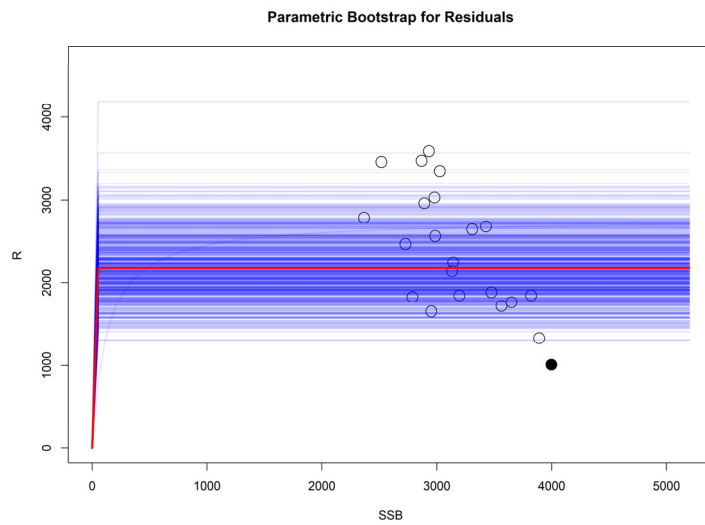
補足図 1-6c. ベバートン・ホルト型再生産関係式を最小二乗法で当てはめた場合の残差ブートストラップ解析の結果
