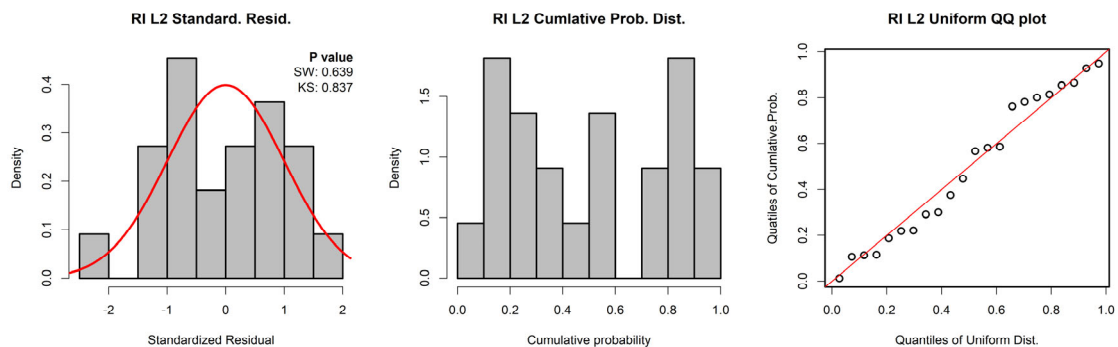
補足図 1-3b. リッカー型再生産関係式を最小二乗法で当てはめた場合の標準化残差のヒストグラムと正規性テスト結果（左図）、残差の累積確率密度のヒストグラム（中央図）、および一様分布を仮定した QQ プロット（右図） 残差のヒストグラムの右上の数値は Shapiro-Wilk 検定（SW）と Kolmogorov-Smirnov 検定（KS）の結果である。どちらも、帰無仮説は「正規分布に従っている」である。QQ プロットの赤線は理論値を示している。
