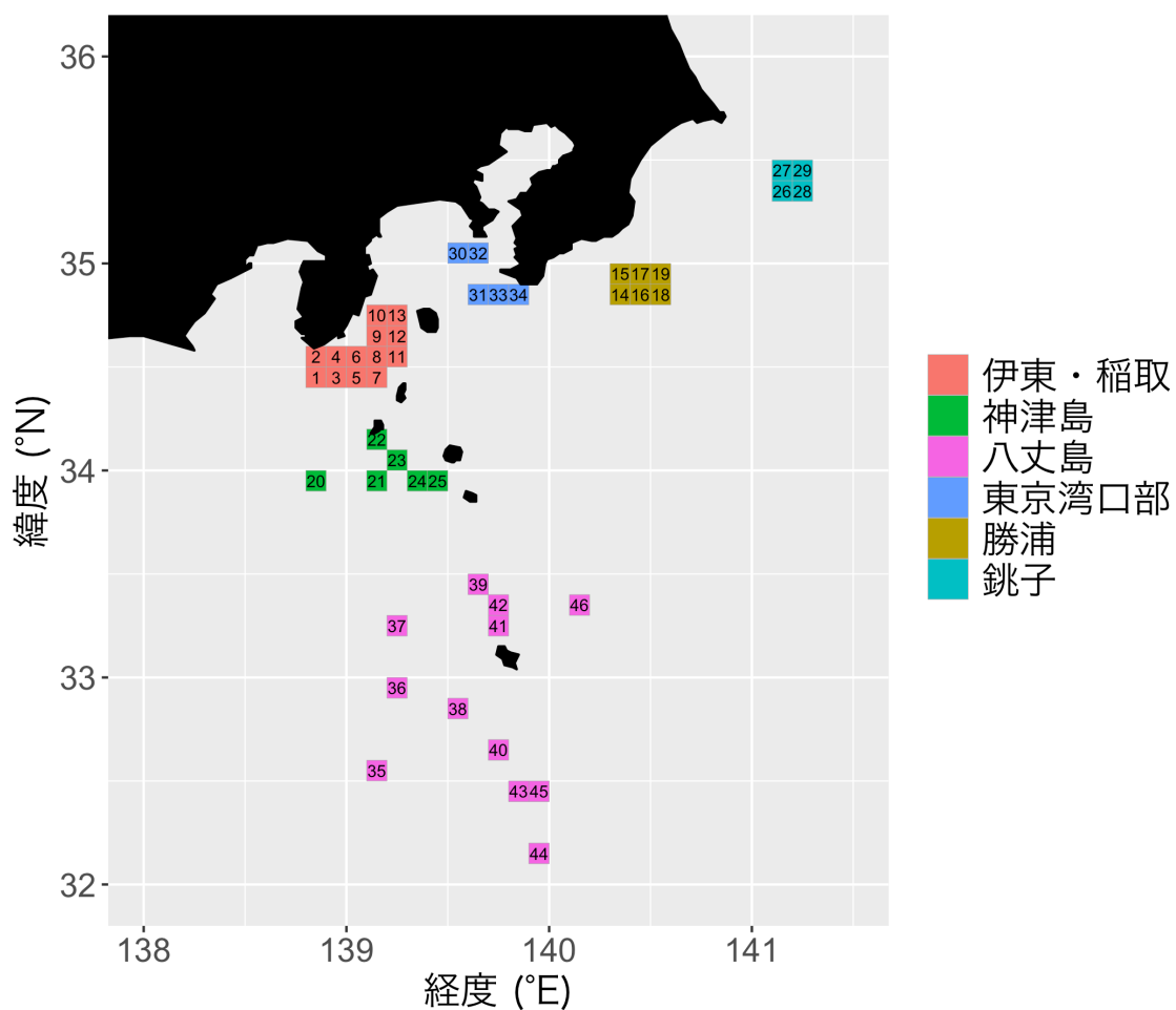
図 1. FRA-ROMS II 再解析値の抽出に用いた各地区の漁場範囲 緯度経度 0.1° グリッドごとにデータを抽出。東京湾口部における千葉県籍船の漁場として、野島崎東側の 33、34 番グリッドを使用。
