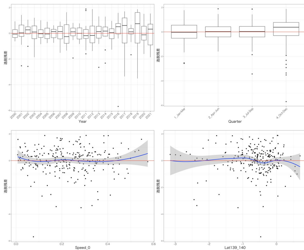
図 6. ベストモデルの層別逸脱残差 Speed_0、Lat139_140 に関する残差図の青線と灰帯は、残差にフィッティングさせた平滑化曲線 (loess) と、その 95%信頼区間を示す。
