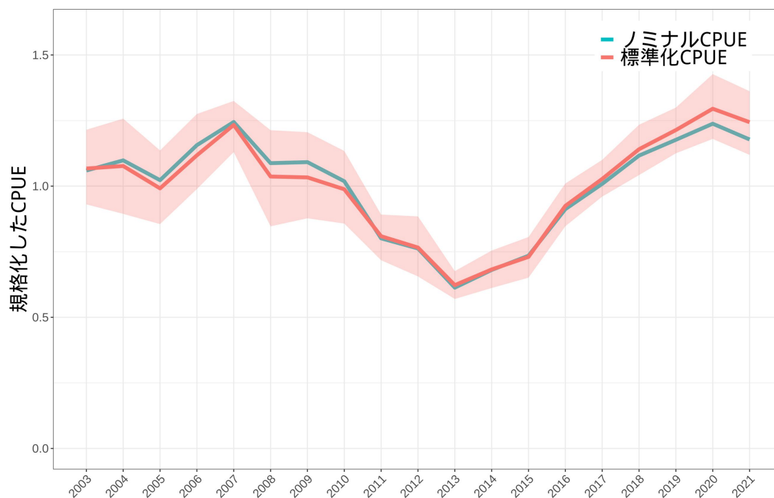
図7. 標準化 CPUE およびノミナル CPUE の推移 赤帯は、データのブートストラップサンプリングとベストモデルによる年トレンド推定を 1000 回繰り返して求めた 95%信頼区間を示す。
