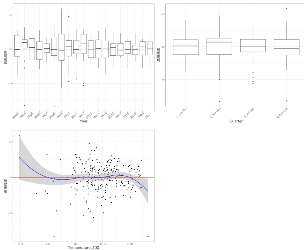
図 6. ベストモデルの層別逸脱残差 Temperature_200 に関する残差図の青線と灰帯は、残差にフィッティングさせた平滑化曲線 (loess) と、その 95%信頼区間を示す。
