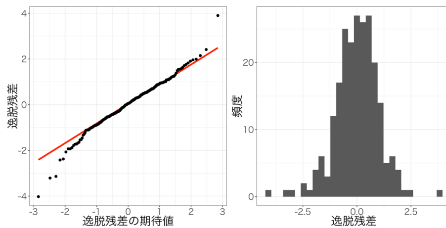
図 5. 各地区のモデルにおける QQ プロット (左) および残差の頻度分布 (右)
