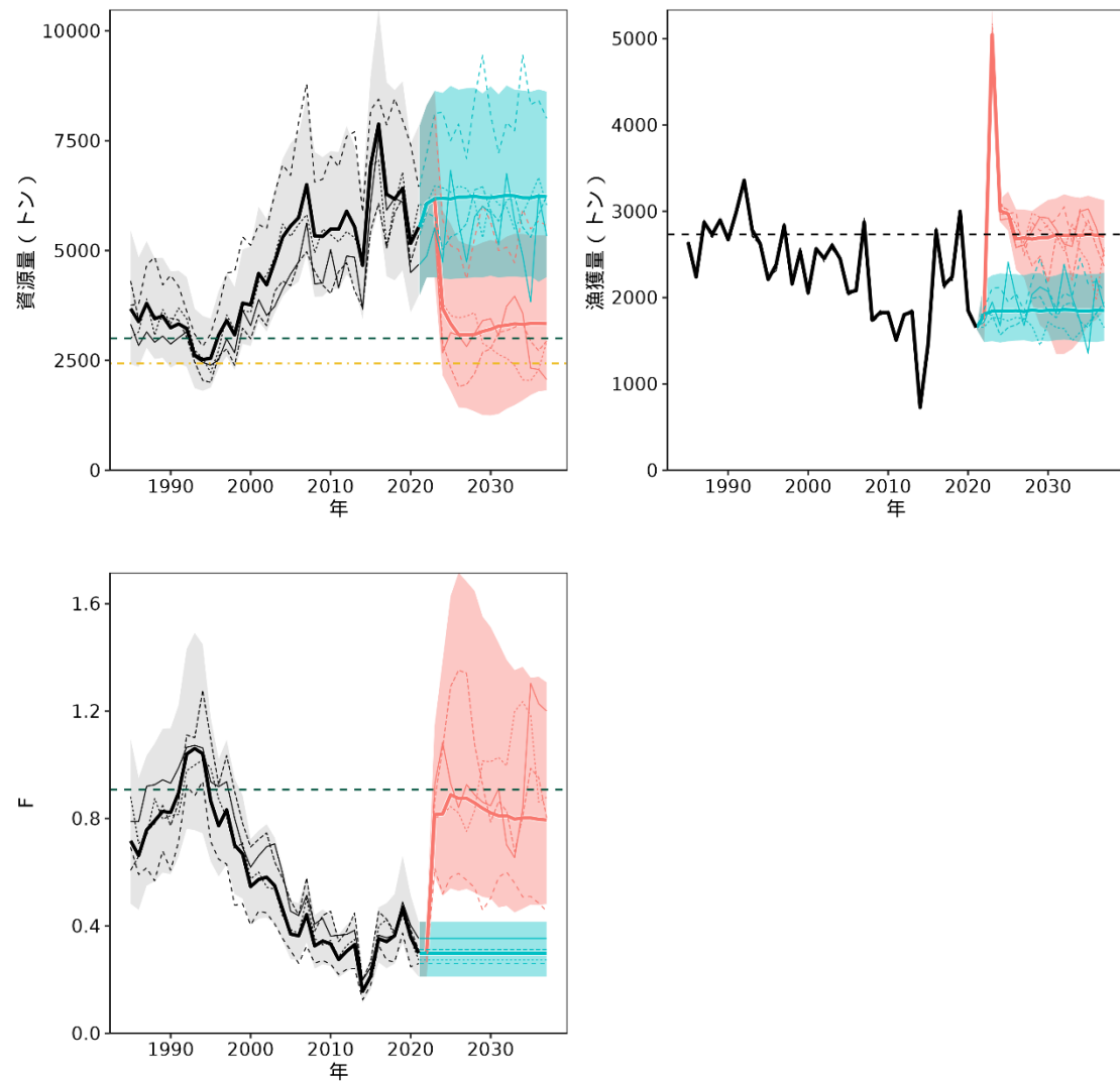
図4. 余剰生産モデルで推定されたパラメータと漁獲管理規則案に基づいて予測された将来の資源量、漁獲圧および漁獲量 青色の太い実線と網掛けは現状の漁獲圧 ( F_{2021} ) で、赤色の太い実線と網掛けは調整係数 \beta=0.8 の漁獲管理規則案で漁獲した場合の予測された値の中央値と 90% 予測区間、黒の太い実線と灰色の網掛けは 2021 年漁期以前の推定された値の中央値と 90% 信頼区間、各色の細い線は反復計算の結果の例示である。緑色の破線は目標管理基準値案を達成する水準、黄色の一点鎖線は限界管理基準値案の水準、漁獲量のパネルに示された黒色の破線は MSY 水準を示す。
