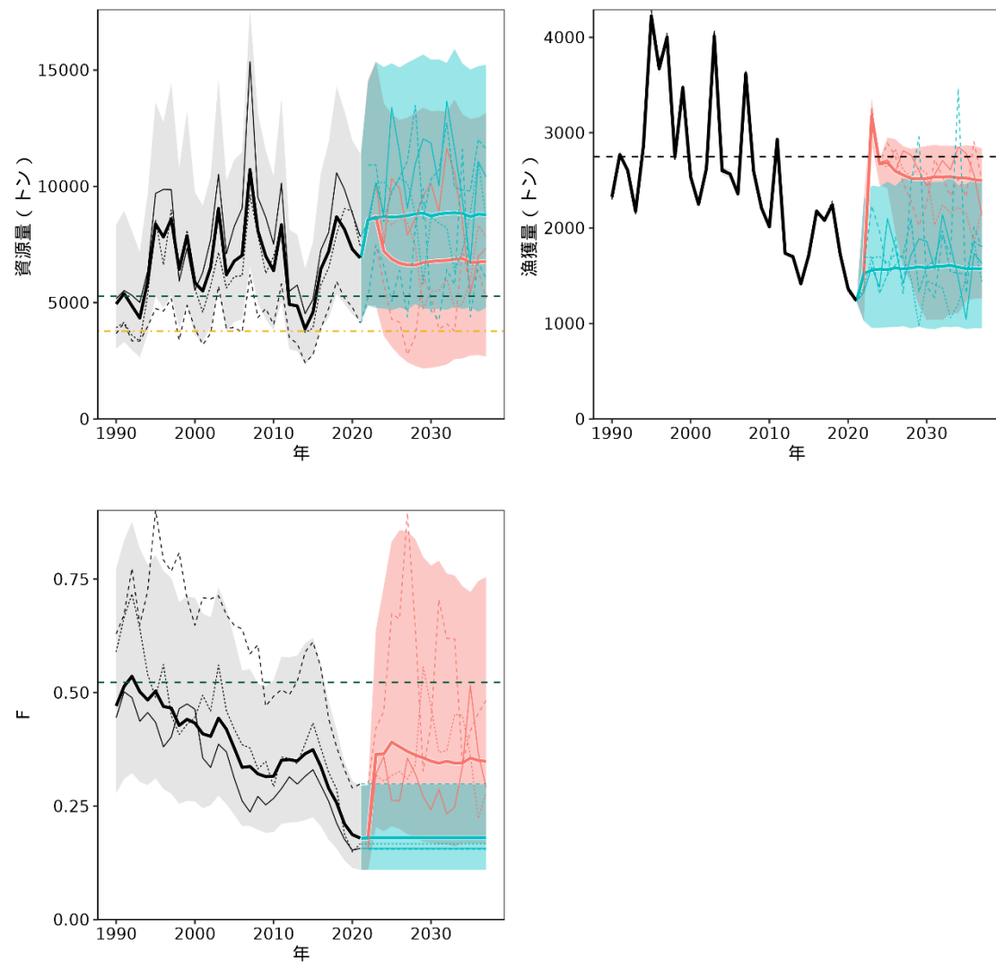
図 4. 余剰生産モデルで推定されたパラメータと漁獲管理規則案に基づいて予測された将来の資源量、漁獲圧および漁獲量 青色の太い実線と網掛けは現状の漁獲圧 ( F_{2021} ) で、赤色の太い実線と網掛けは調整係数 \beta=0.7 の漁獲管理規則案で漁獲した場合の予測された値の中央値と 90% 予測区間、黒の太い実線と灰色の網掛けは 2021 年漁期以前の推定された値の中央値と 90% 信頼区間、各色の細い線は反復計算の結果の例示である。緑色の破線は目標管理基準値案を達成する水準、黄色の一点鎖線は限界管理基準値案の水準、漁獲量のパネルに示された黒色の破線は MSY 水準を示す。
