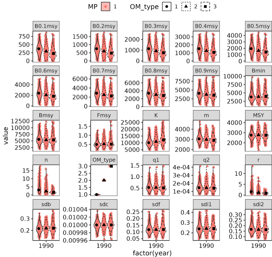
補足図3 将来予測用に再生成したパラメータセットの分布
