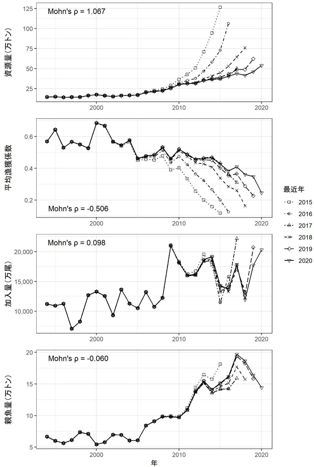
図 5. レトロスペクティブ解析 (従来 VPA)
