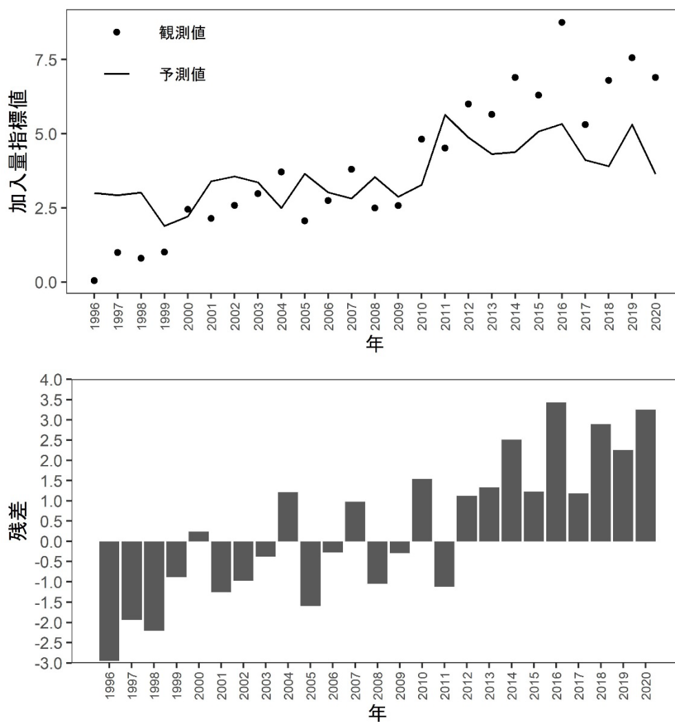
図3. チューニング VPA による加入量指標の予測値と観測値の推移（上段）と残差（下段）の推移
