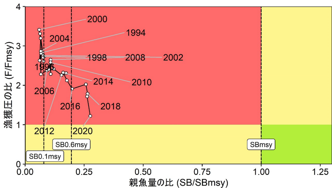
図 8. 神戸プロット
