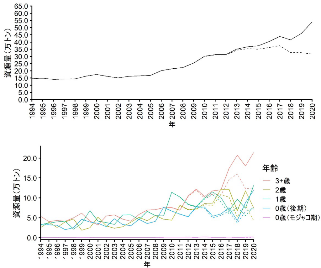
図 1. チューニング VPA による資源評価結果への影響 (資源量)
