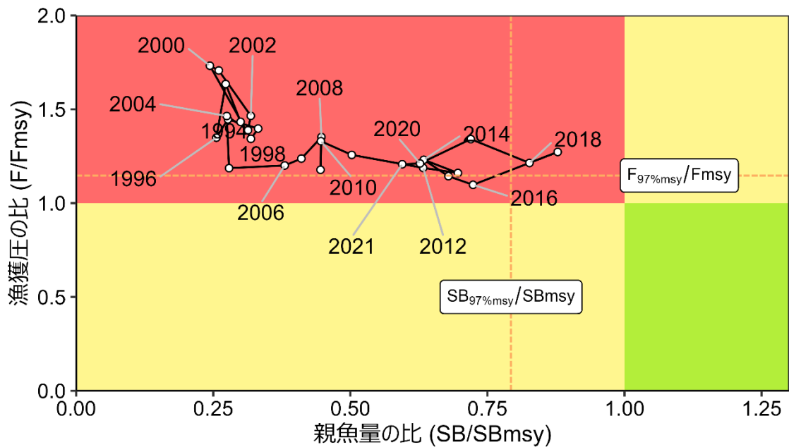
図 2. 神戸プロット 橙破線は、SBmsy と Fmsy に対する、97%MSY を達成することが期待できる親魚量 (SB97%msy) および漁獲圧 (F97%msy) の比をそれぞれ示す。
