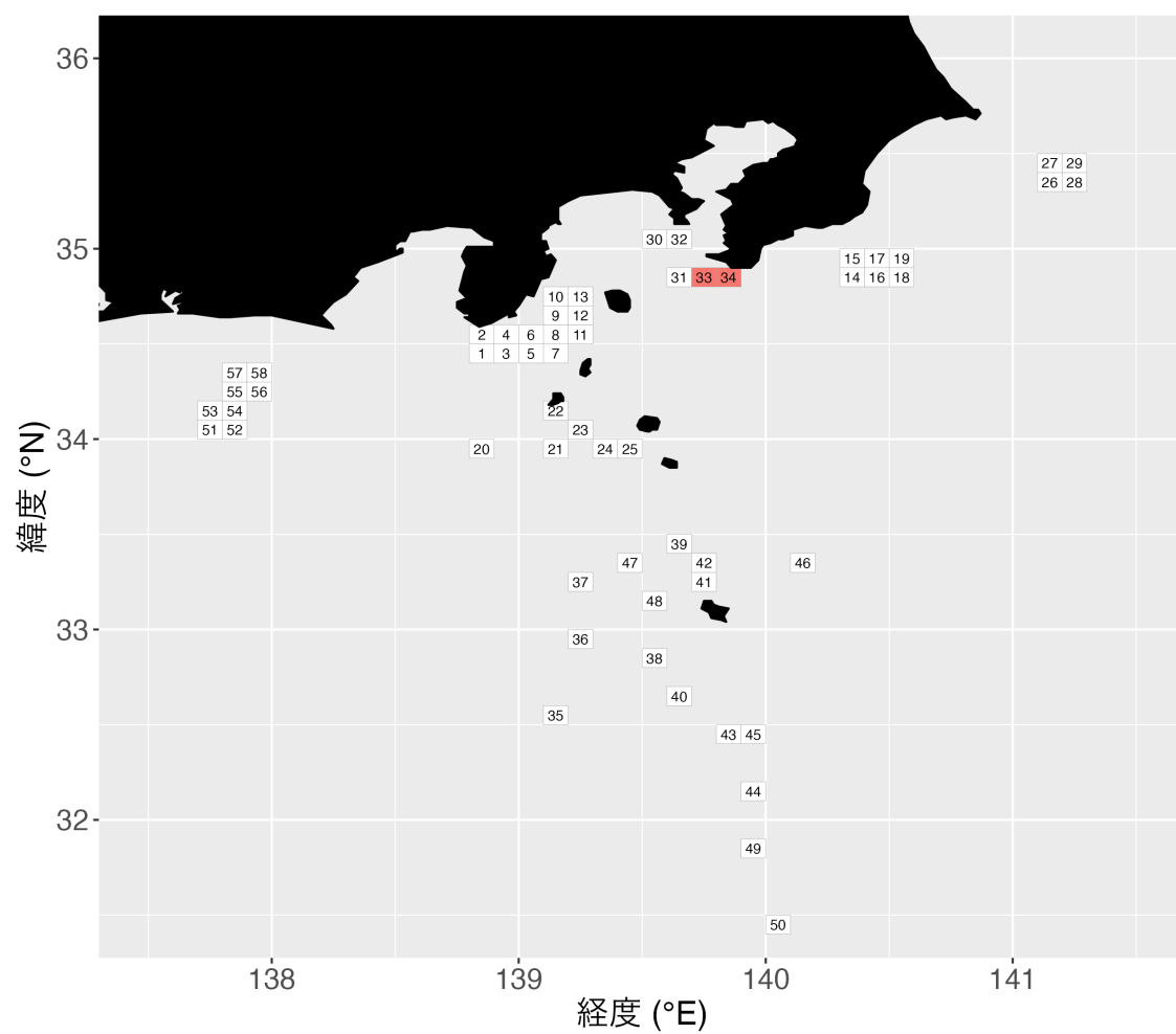
図 1. FRA-ROMS II再解析値の抽出を行う漁場位置の候補 緯度経度 0.1°グリッドごとにデータを抽出。東京湾口部は 33、34 番のグリッドを使用。
