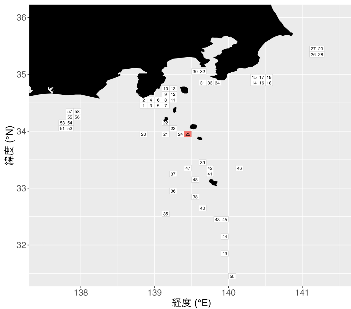
図 1. FRA-ROMS II再解析値の抽出を行う漁場位置の候補 緯度経度 0.1°グリッドごとにデータを抽出。三宅島地区は 25 番のグリッドを使用。
