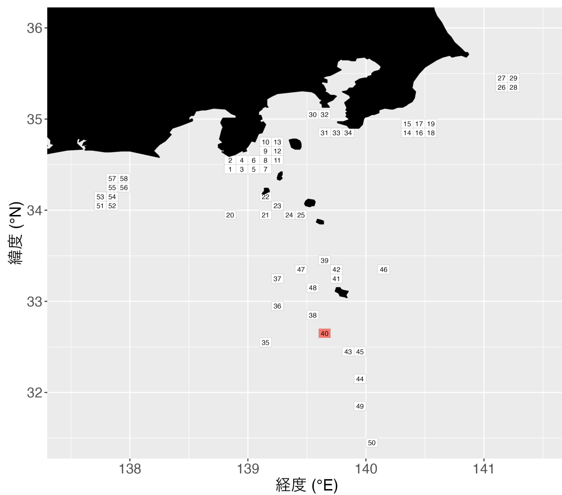
図 1. FRA-ROMS II再解析値の抽出を行う漁場位置の候補 緯度経度 0.1°グリッドごとにデータを抽出。八丈島地区は 40 番のグリッドを使用。
