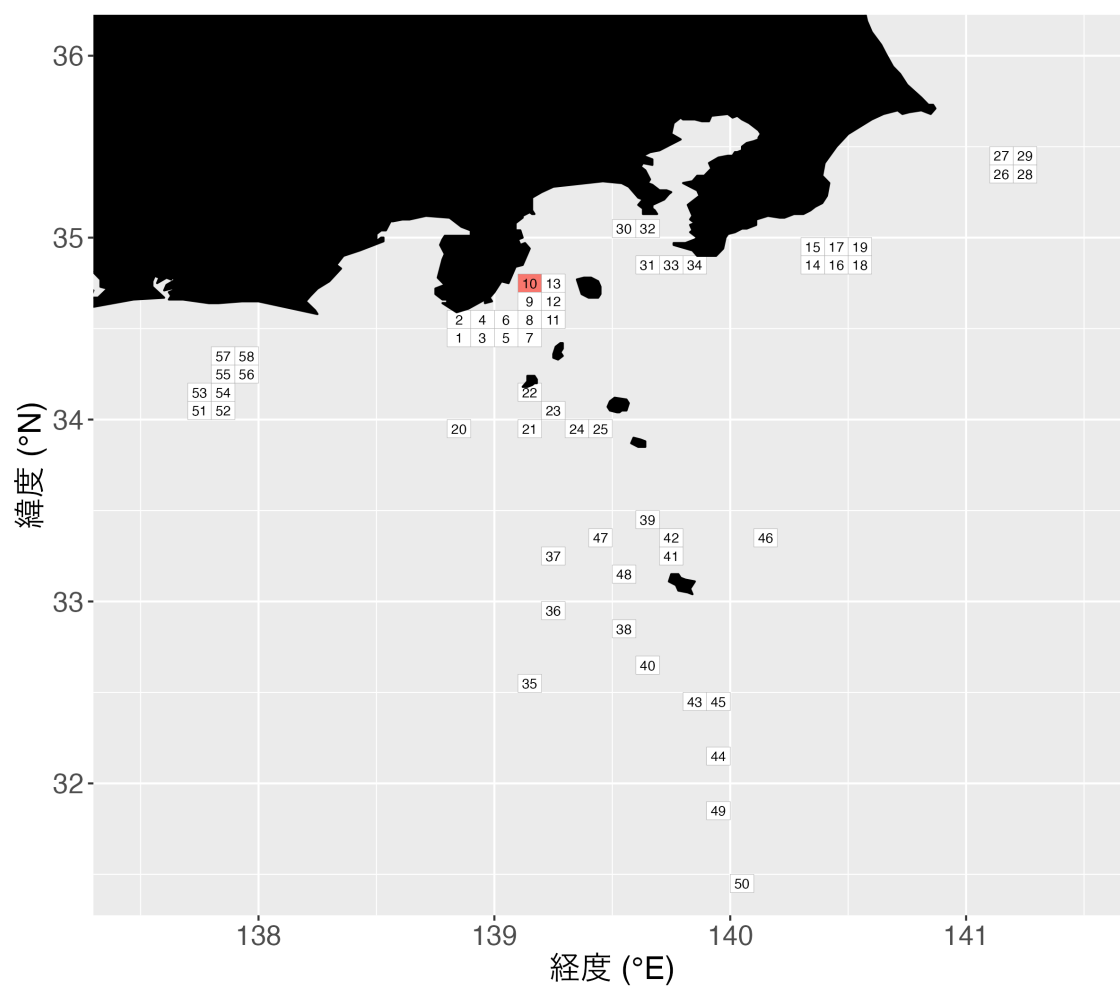
図 1. FRA-ROMS II再解析値の抽出を行う漁場位置の候補 緯度経度 0.1°グリッドごとにデータを抽出。伊東地区は 10 番のグリッドを使用。
